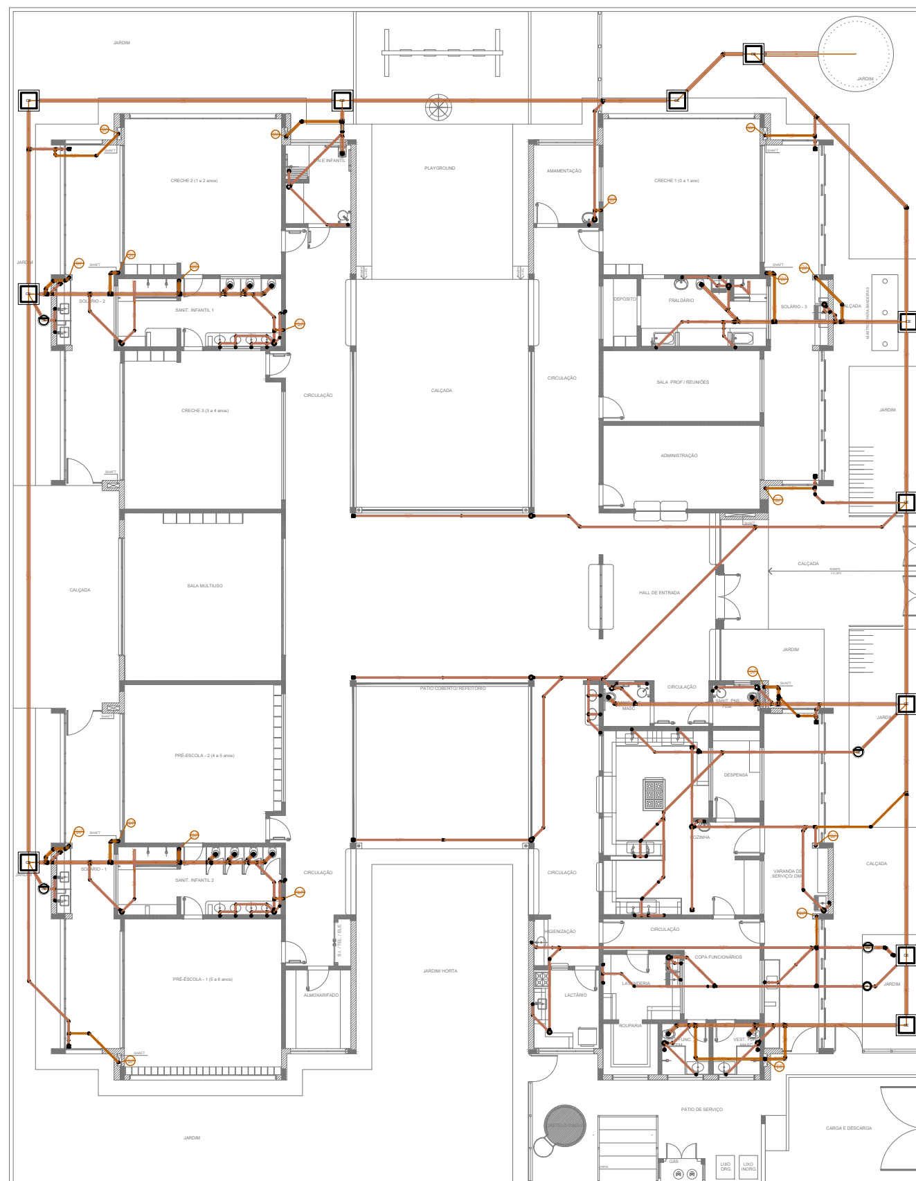
9 PLANTA BAIXA - ESGOTO TUBULAÇÕES EXISTENTES ESCALA 1/200
