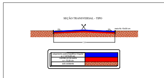
DETALHAMENTO DE SEÇÃO TRANSVERSAL ESCALA 1/50
