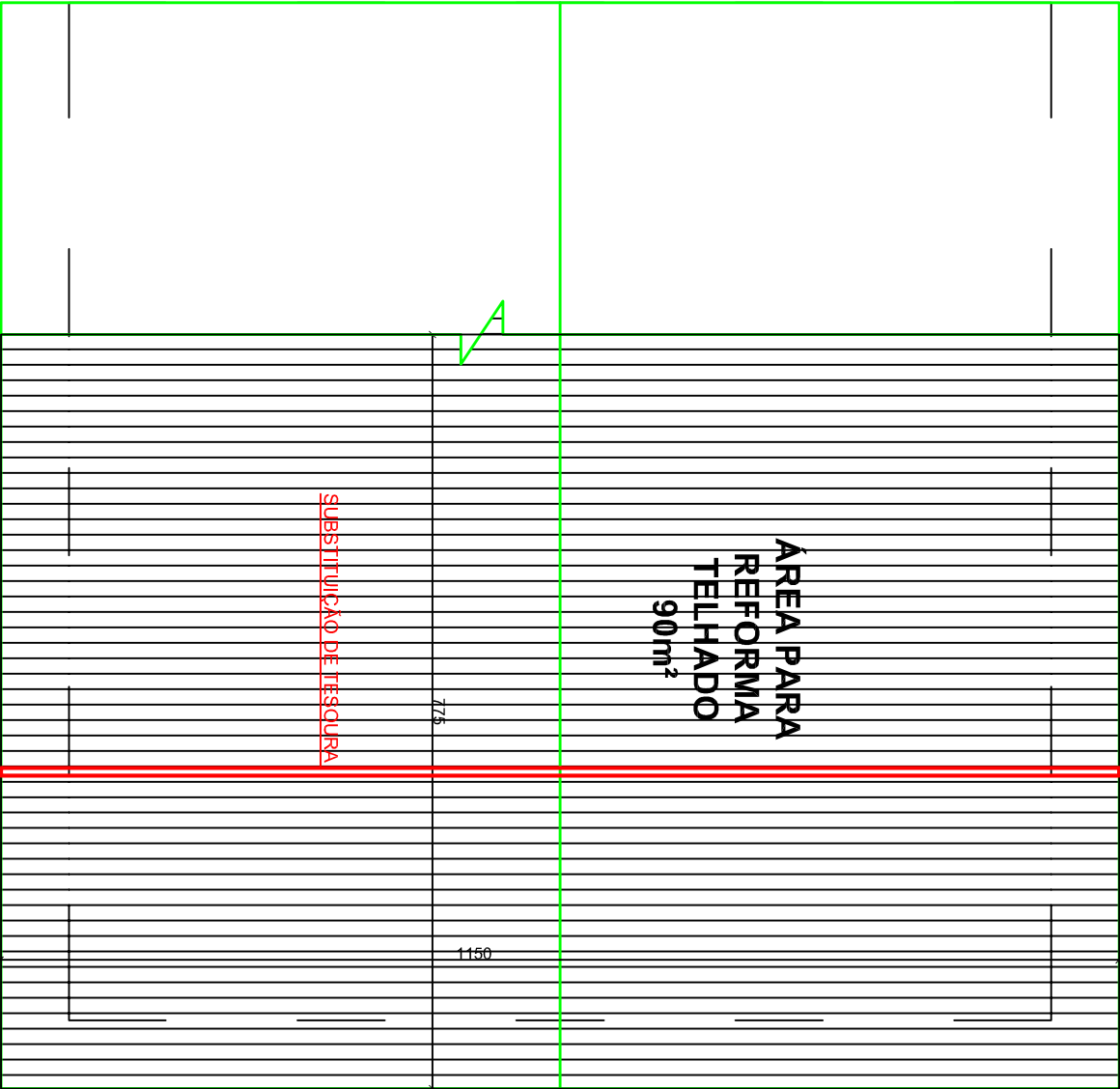
PLANTA DE SERVIÇOS A SEREM EXECUTADOS - COBERTURA
