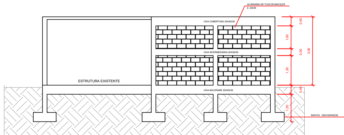
04 VISTA FRENTE MURO
