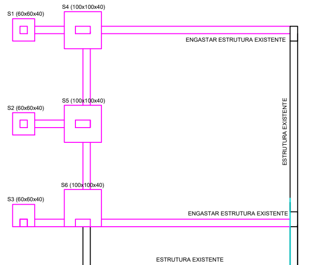
01 PLANTA DE FORMAS FUNDAÇÕES
