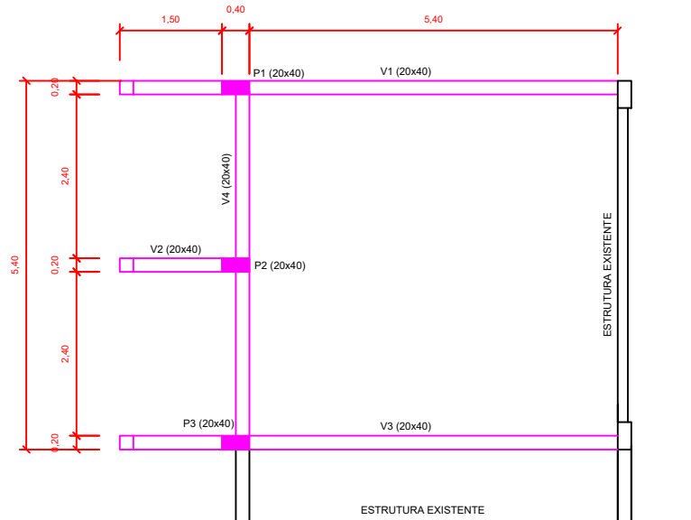
02 PLANTA DE FORMAS BALDRAME
