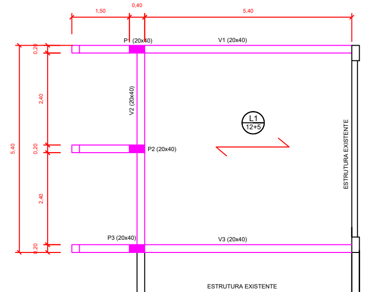
03 PLANTA DE FORMAS COBERTURA
