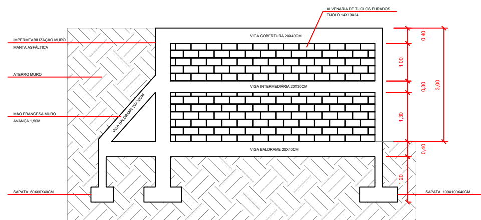
05 VISTA LATERAL MURO
