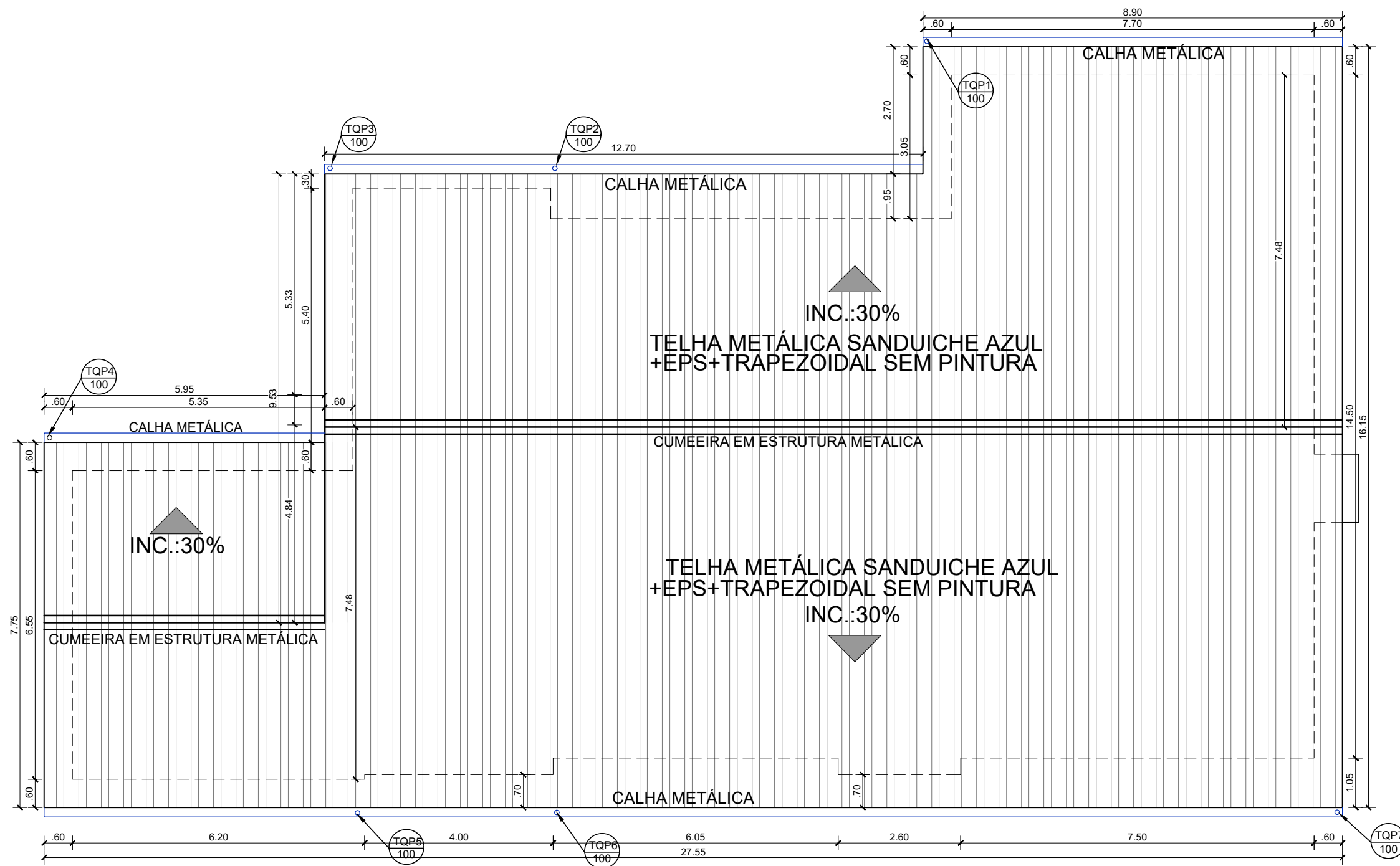
04 PLANTA DE COBERTURA 2 ESCALA 1/100 ÁREA DO TELHADO: 361M 2
