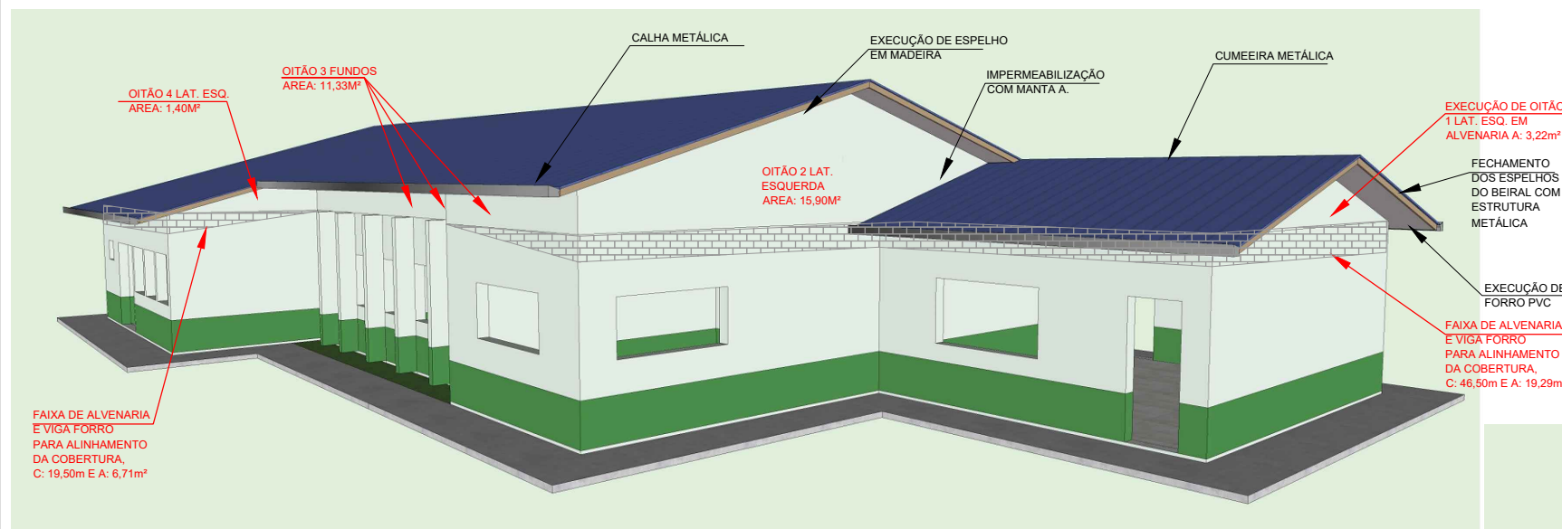
05 PERSPECTIVA 1
