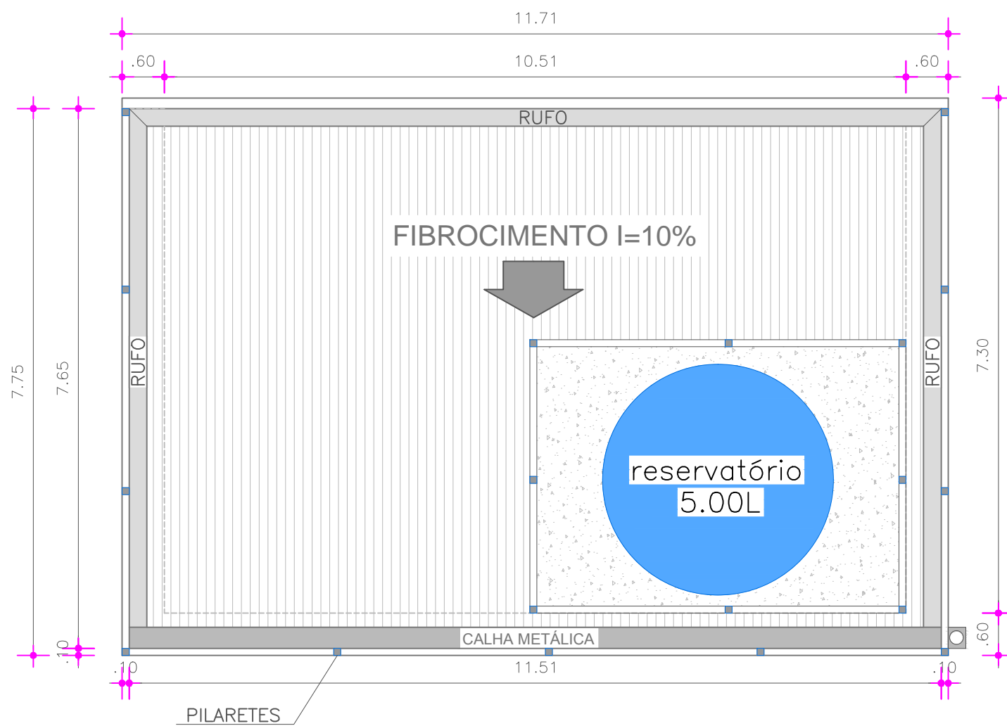
01 Cobertura ESCALA: 1/75
