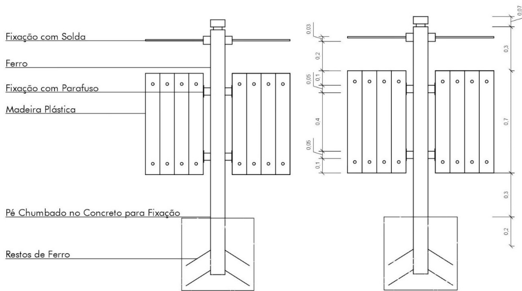
VISTA LATERAL
