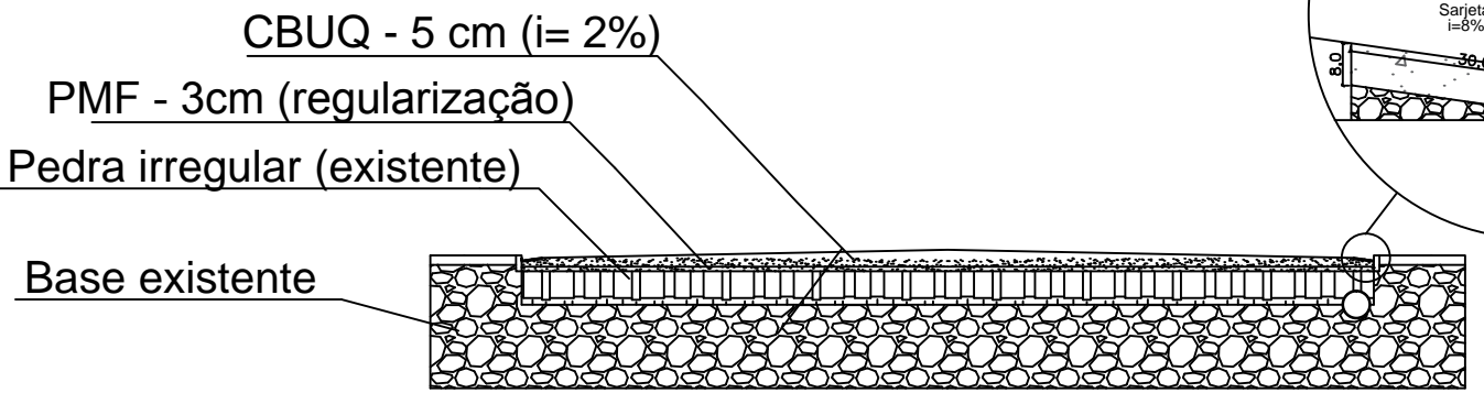
○ CORTE A-A ESCALA: 5/ESCALA
