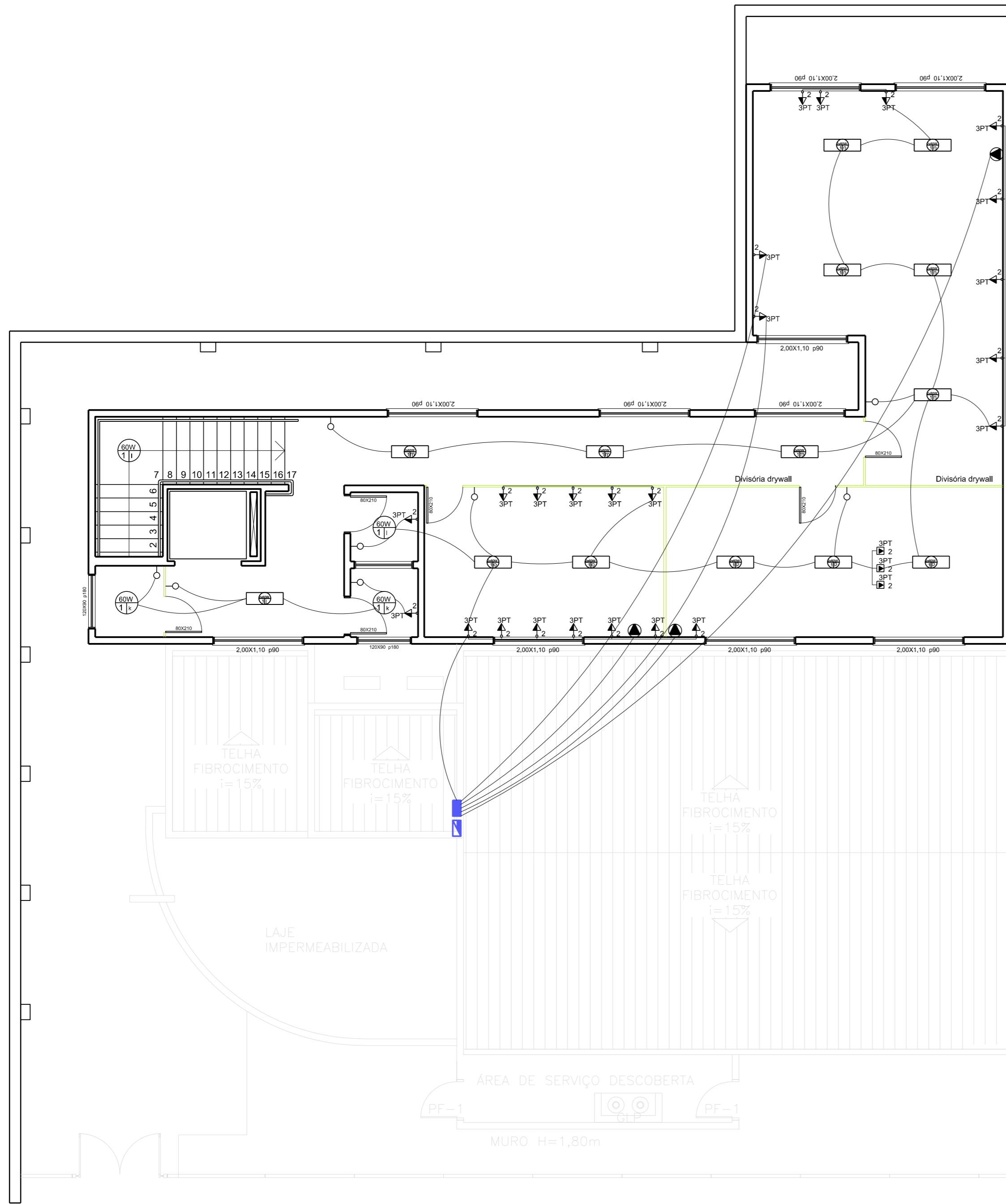
PLANTA COBERTURA CRAS PORTE I E II ÁREA: 165,30 m 2
