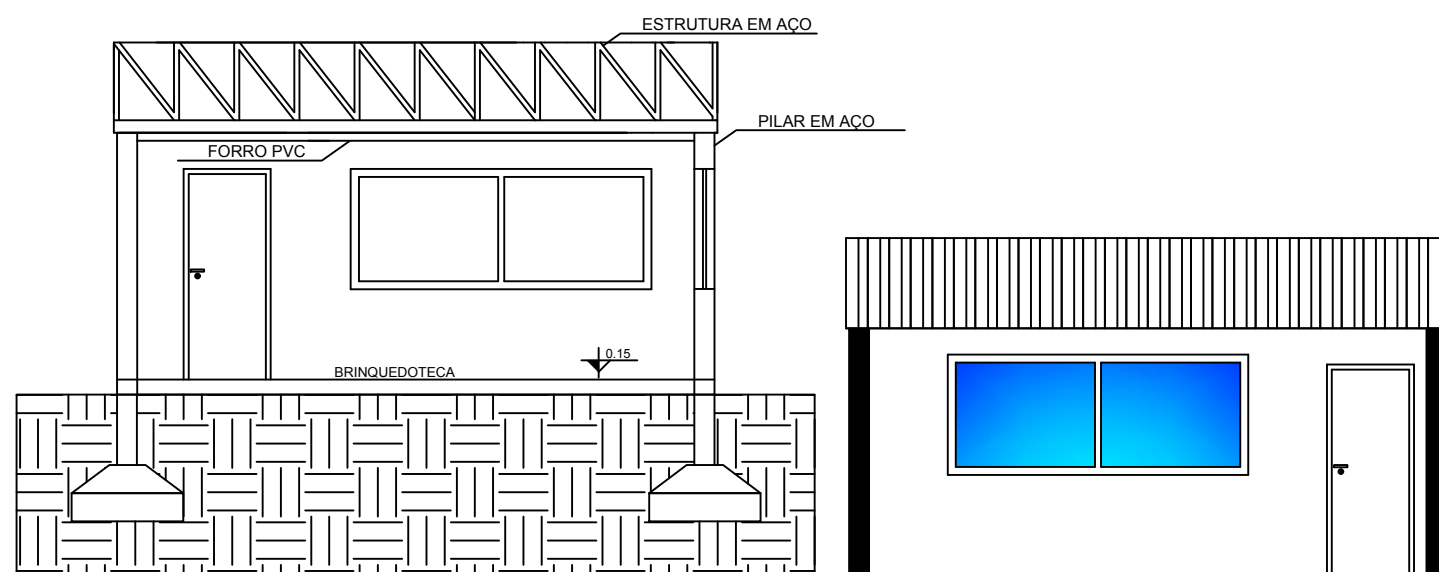
01 CORTE A-A'
