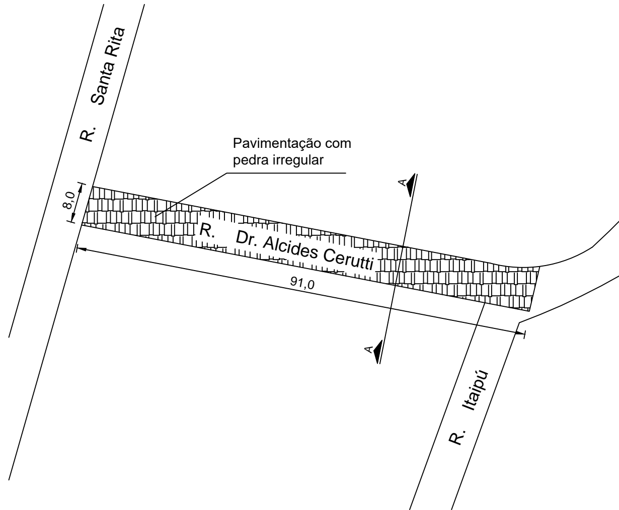
PLANTA BAIXA ÁREA: 728,0 m 2
