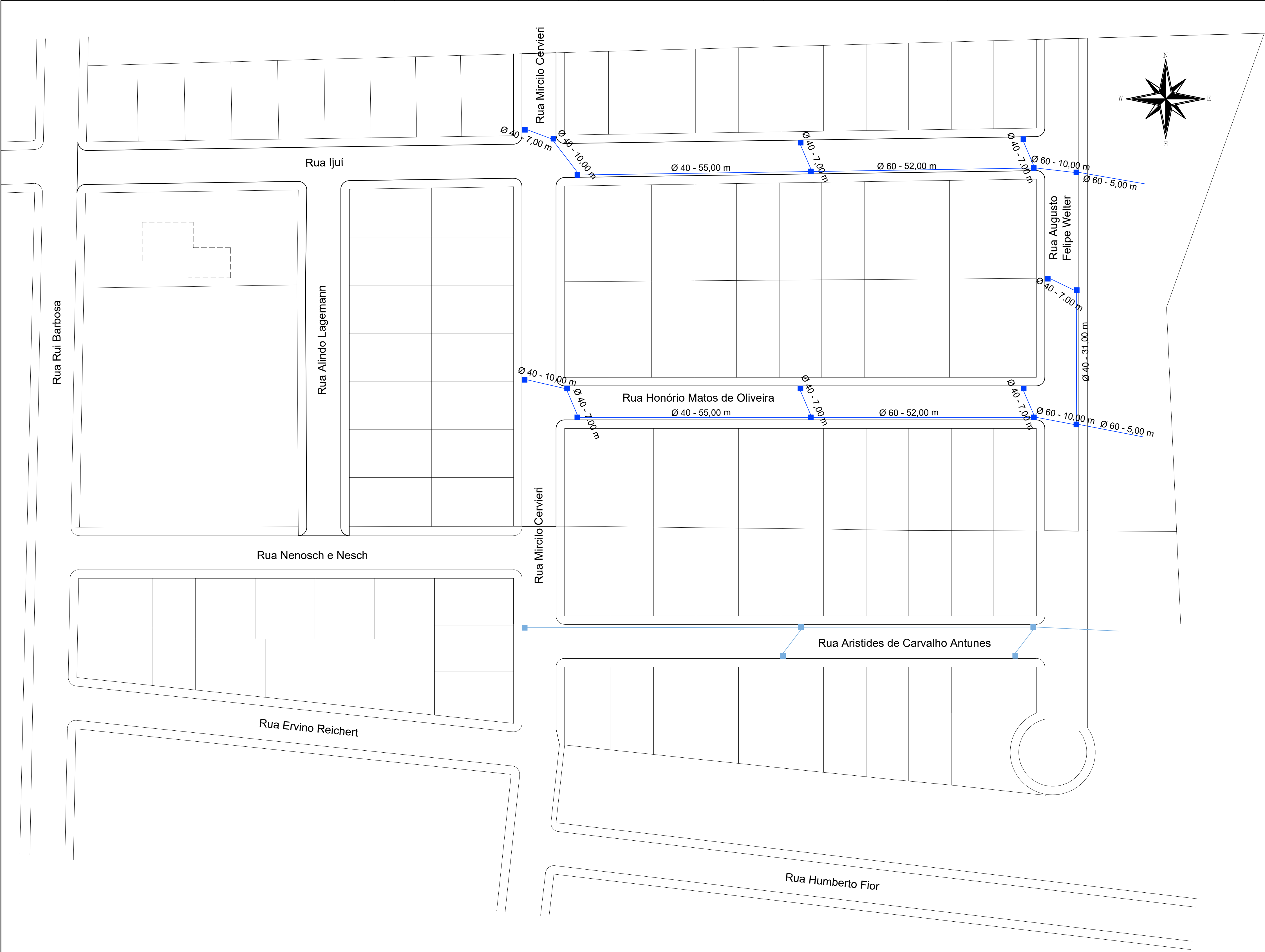
PROJETO DE DRENAGEM Escala 1:500
