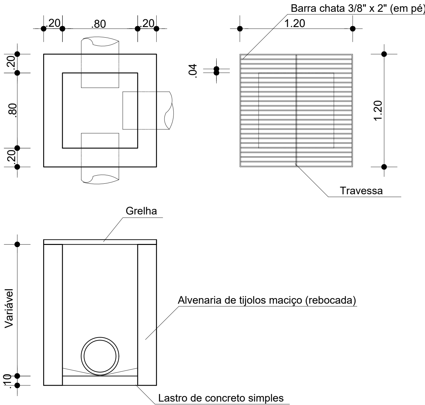
BOCA DE LOBO 1.20 X 1.20 Escala 1:25
