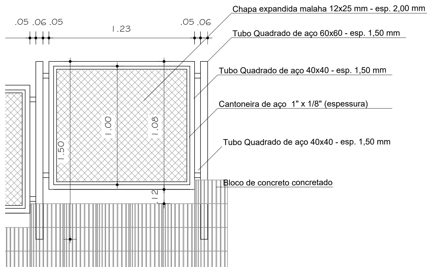
DETALHE 01 Escala: 1/20
