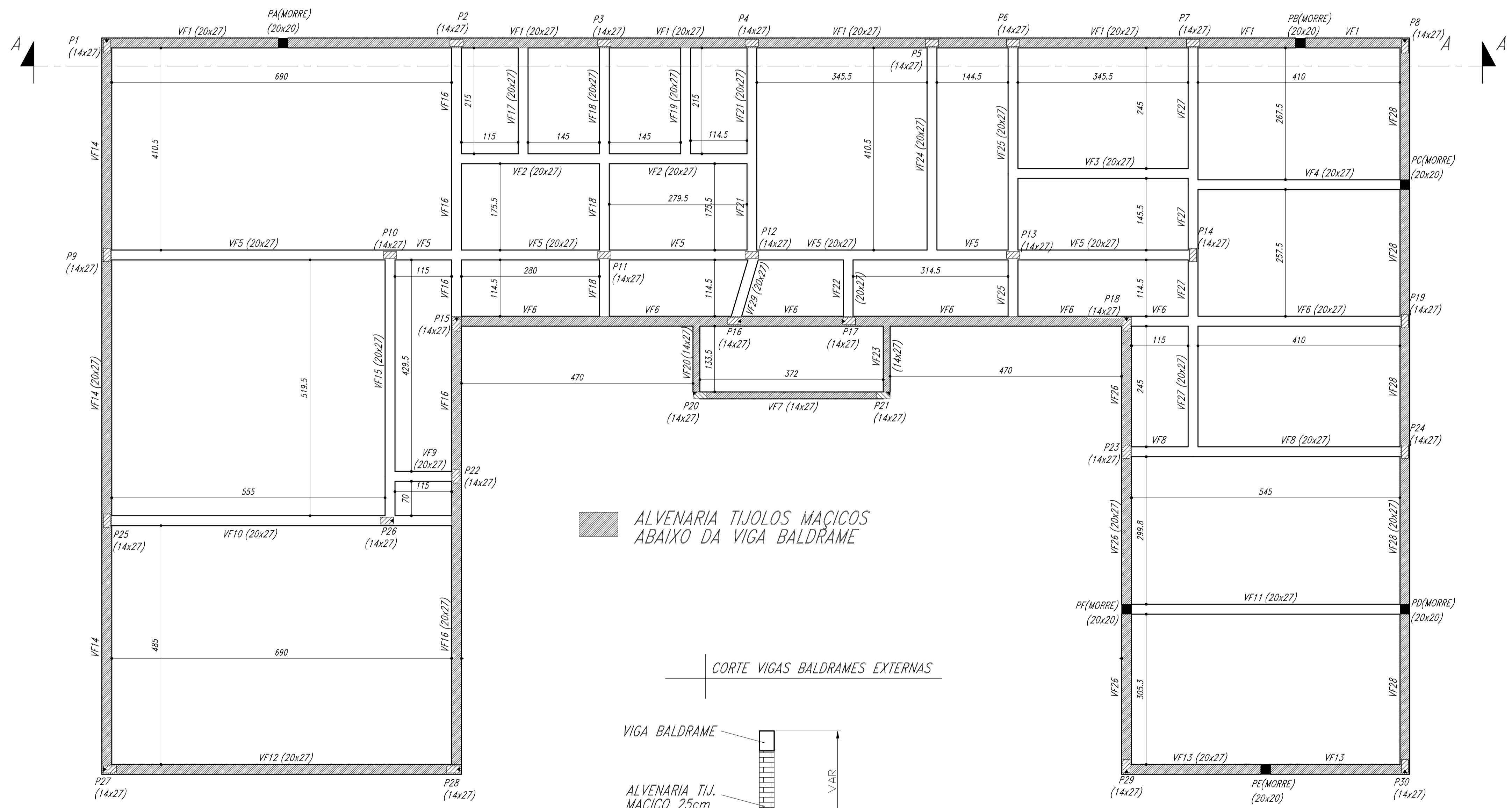
Forma do pavimento FUNDAÇÃO (Nível 0) escala 1:50
