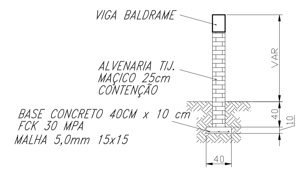
CORTE VIGAS BALDRAMES EXTERNAS
