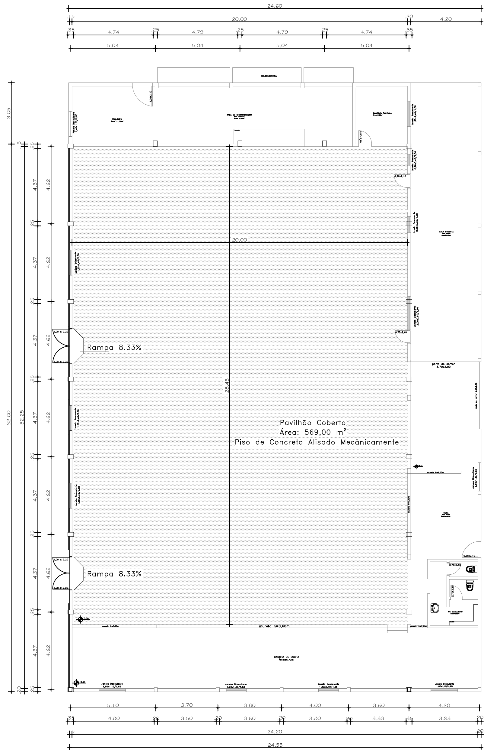
PLANTA BAIXA Escala: 1/125
