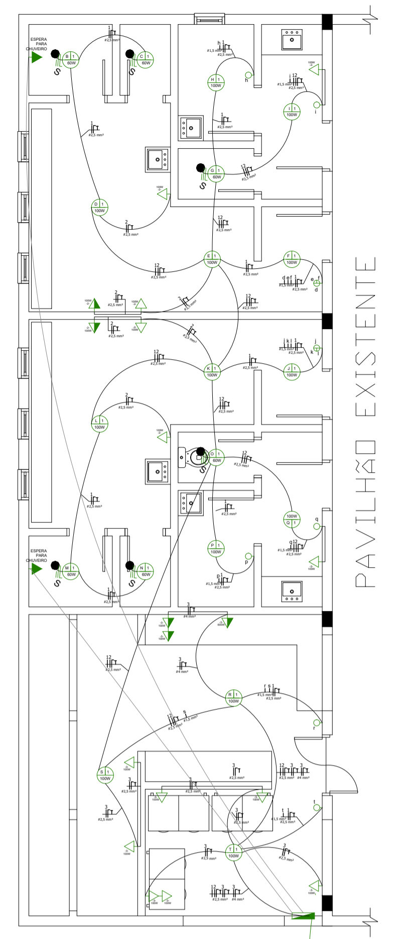
PROJETO ELÉTRICO Escala 1/100
