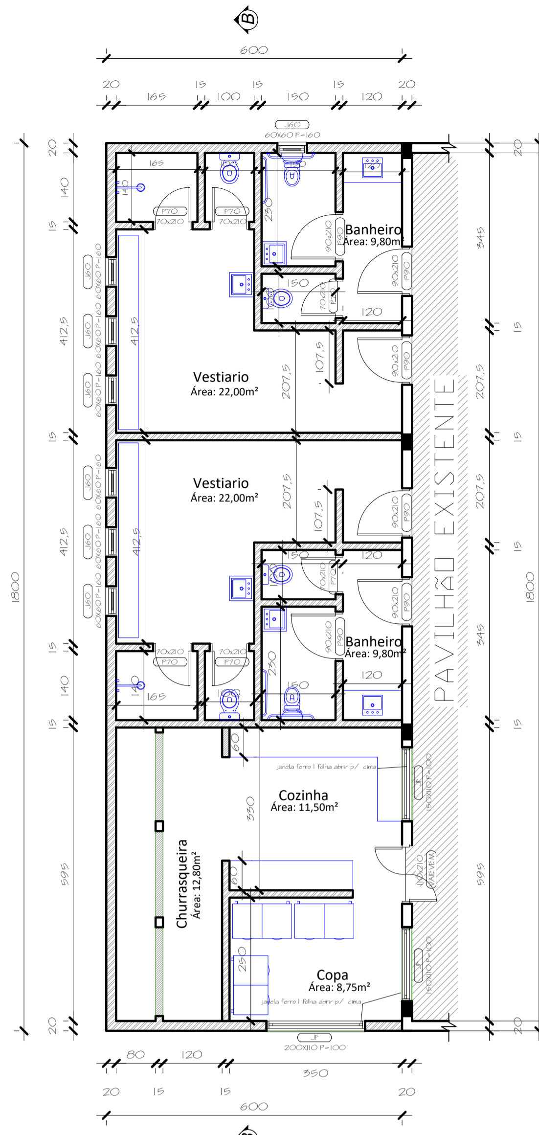
PLANTA BAIXA Escala 1/100
