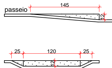
DETALHE RAMPAS
