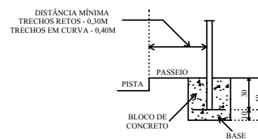
DETALHE FIXAÇÃO SINALIZAÇÃO LOGRADOUROS DIVERSOS
