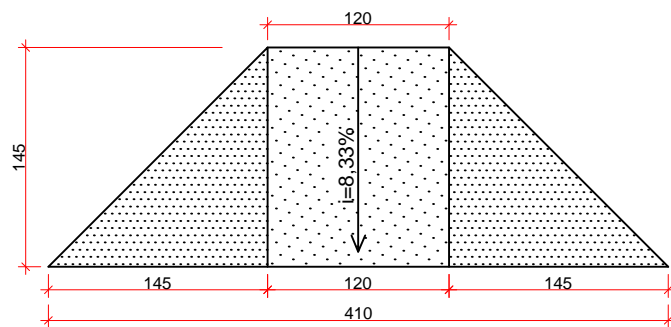
DETALHE RAMPAS
