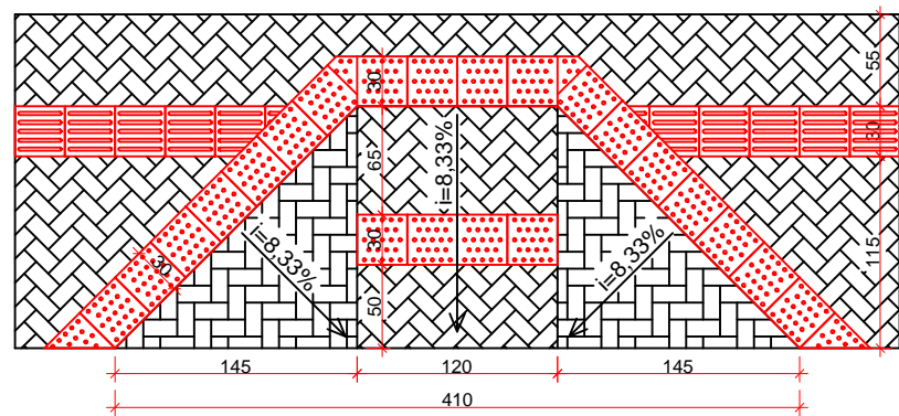
DETALHE RAMPAS SINALIZAÇÃO TÁTIL DIRECIONAL E ALERTA
