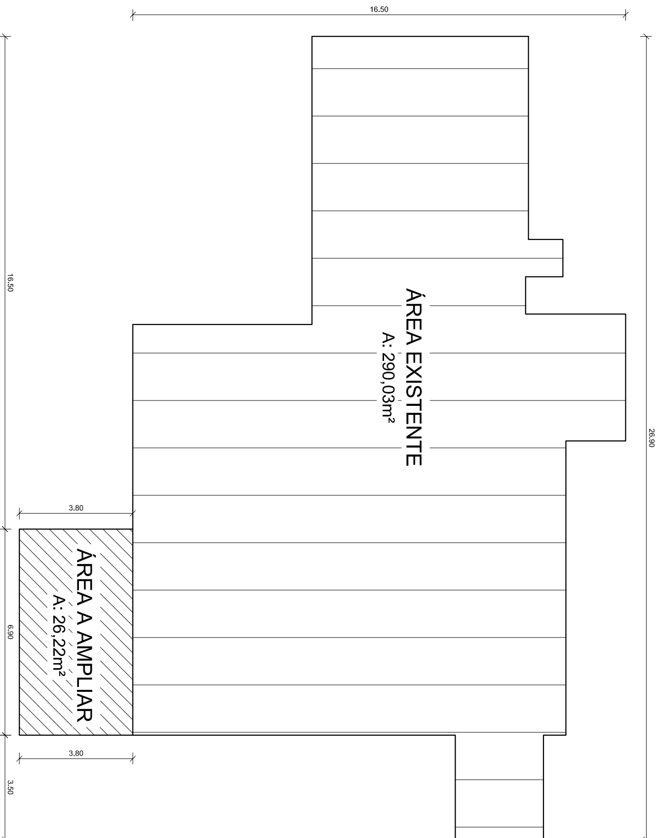
PLANTA DE LOCALIZAÇÃO Escala: 1/125
