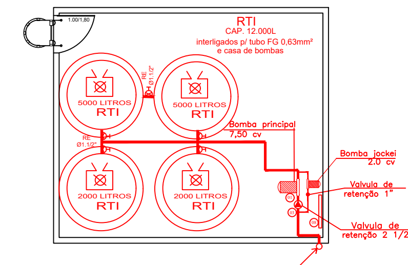
PL. BXA CASA DE MAQUINAS ESCALA: 1:100
