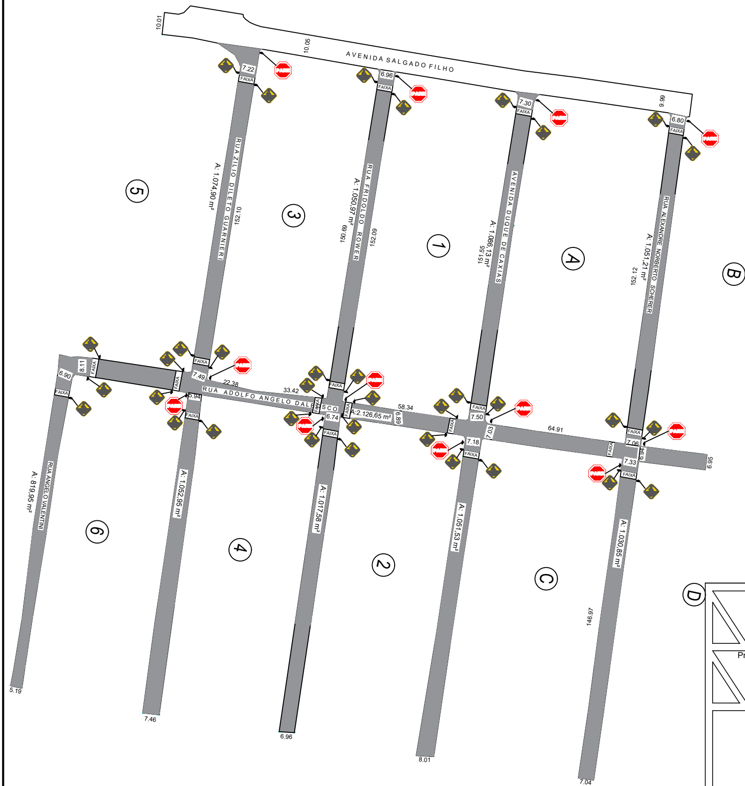
01 Planta de planificação 1/100
