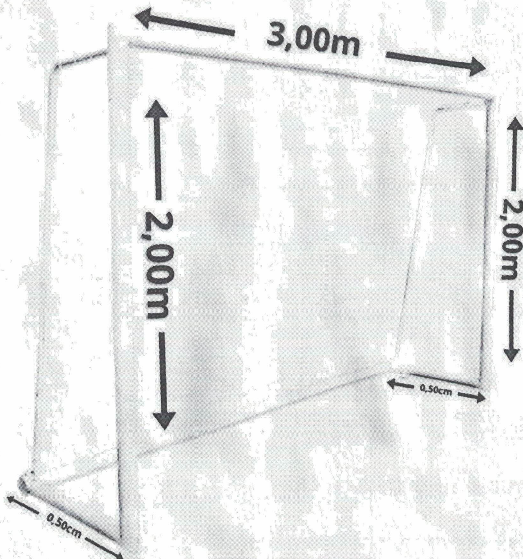
Figura 2 - Dimensões Goleiras
