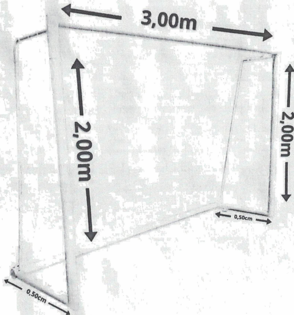
Figura 2 - Dimensões Goleiras
