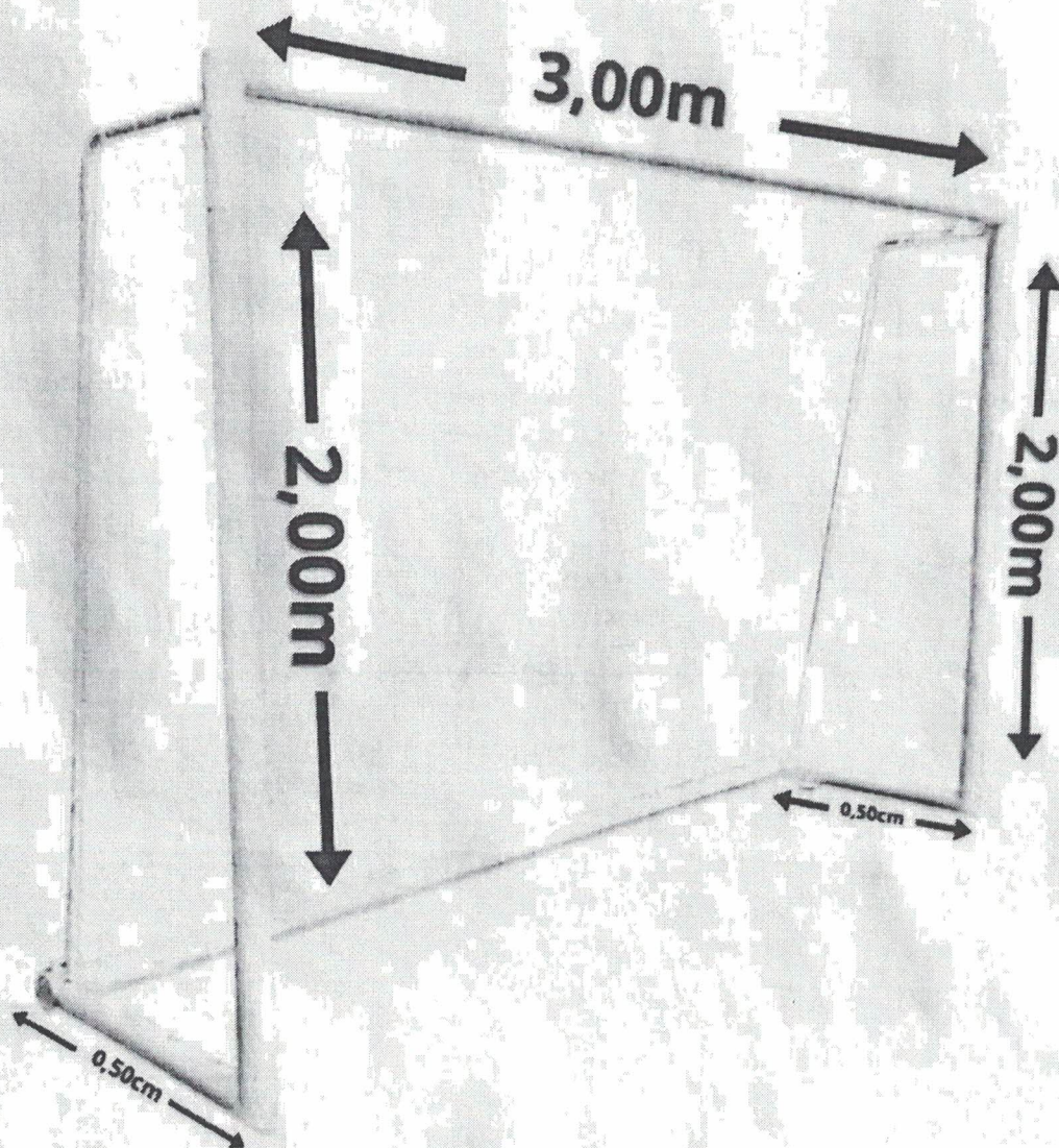
Figura 2 - Dimensões Goleiras
