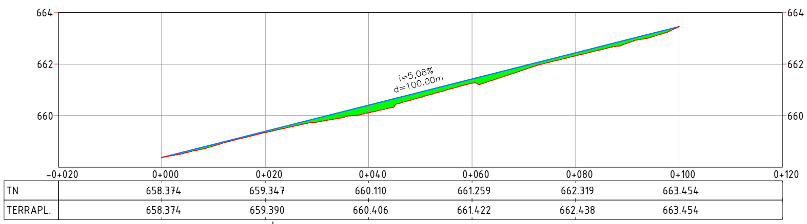
PERFIL LONGITUDINAL RUA DOS DESPORTOS | ESCALA HORIZONTAL: 1:200 / ESCALA VERTICAL: 1:40
