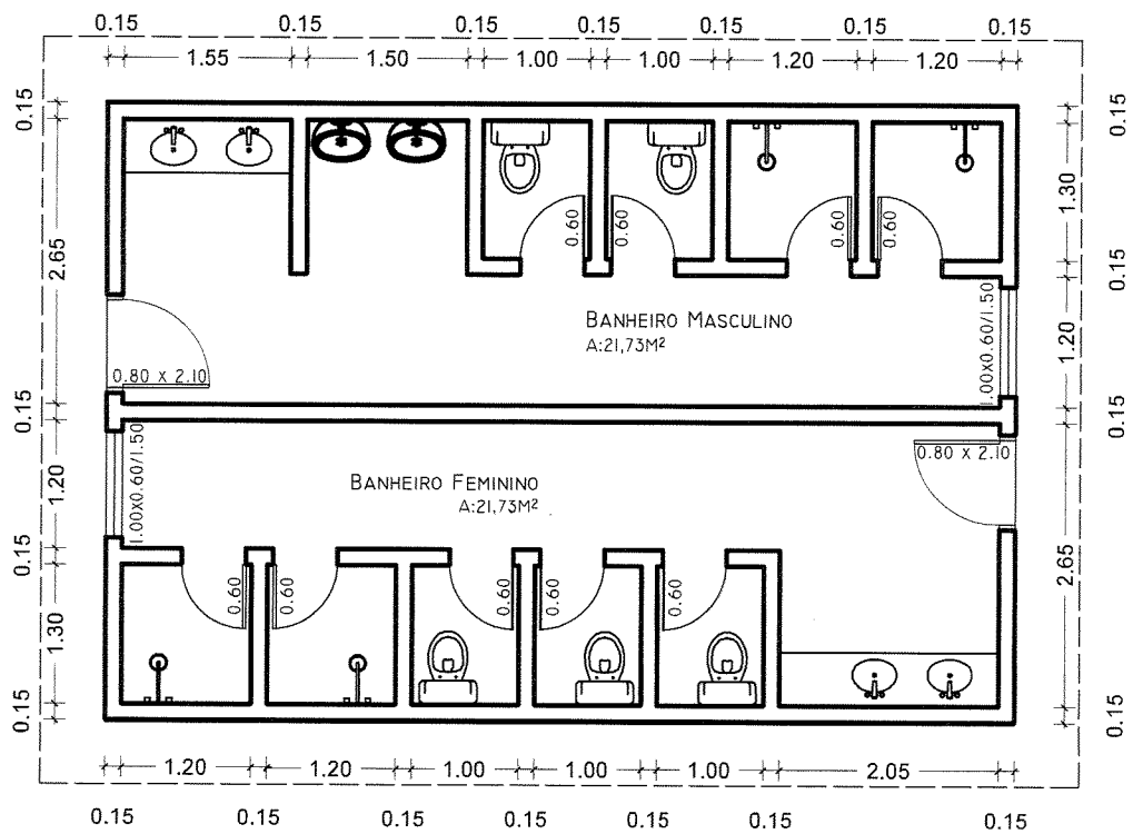
1 PLANTA BAIXA BANHEIROS A: 48,87M 2
