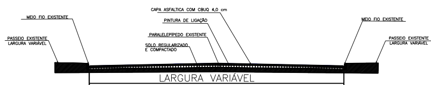
SEÇÃO TIPO
