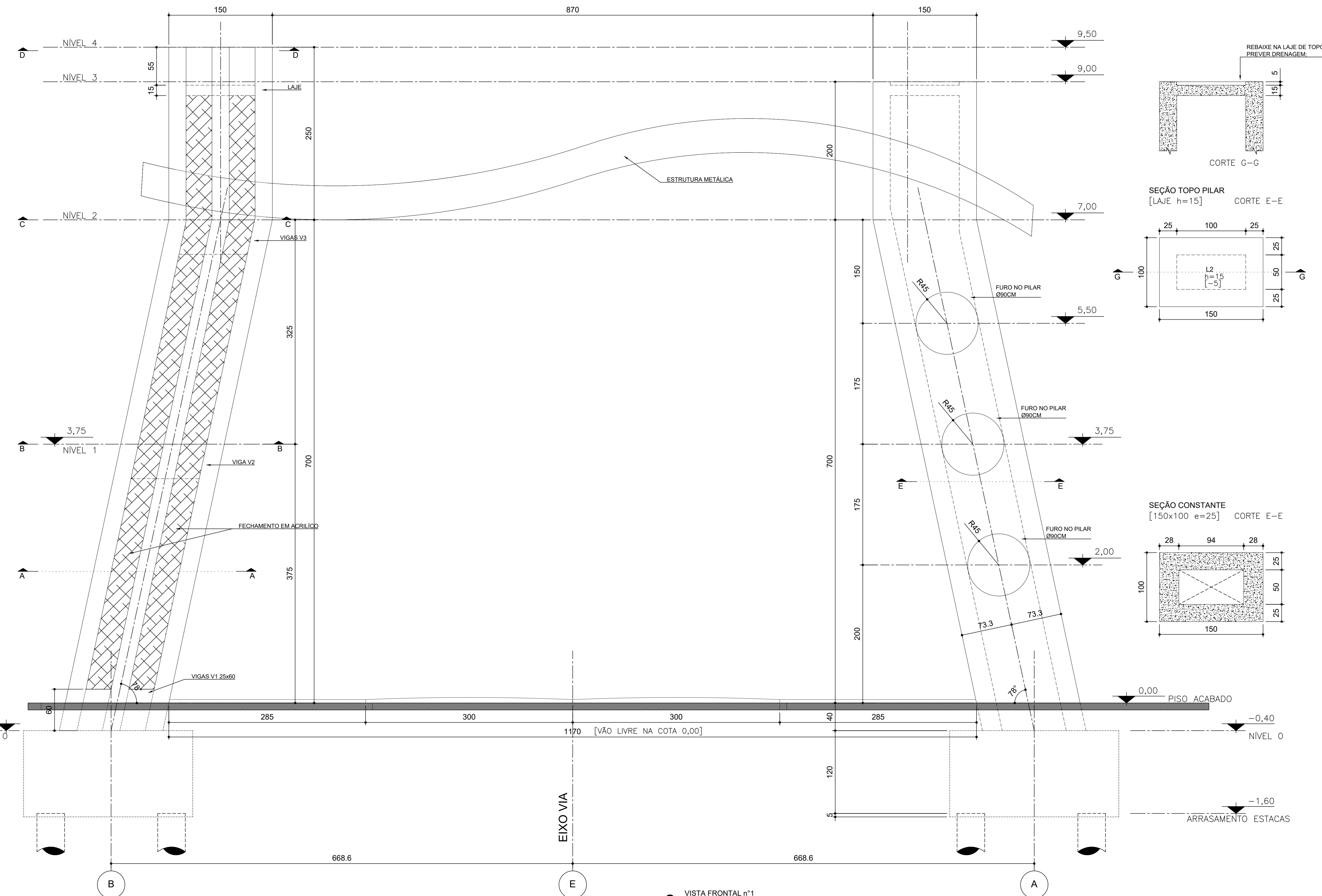
VISTA FRONTAL n°1 esc.: 1/25 [cm]
