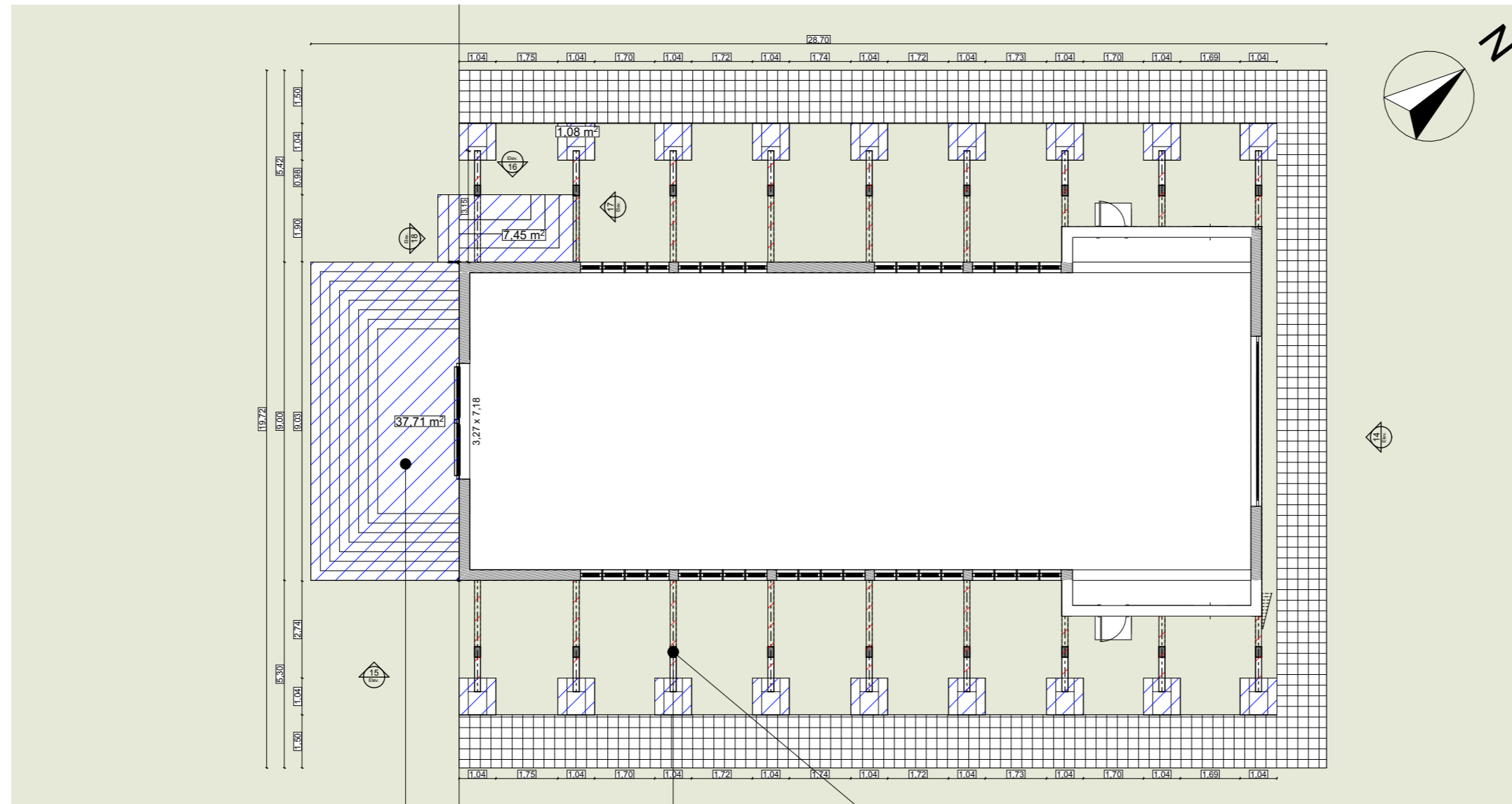
Planta de Intervenções Esc. 1:150
