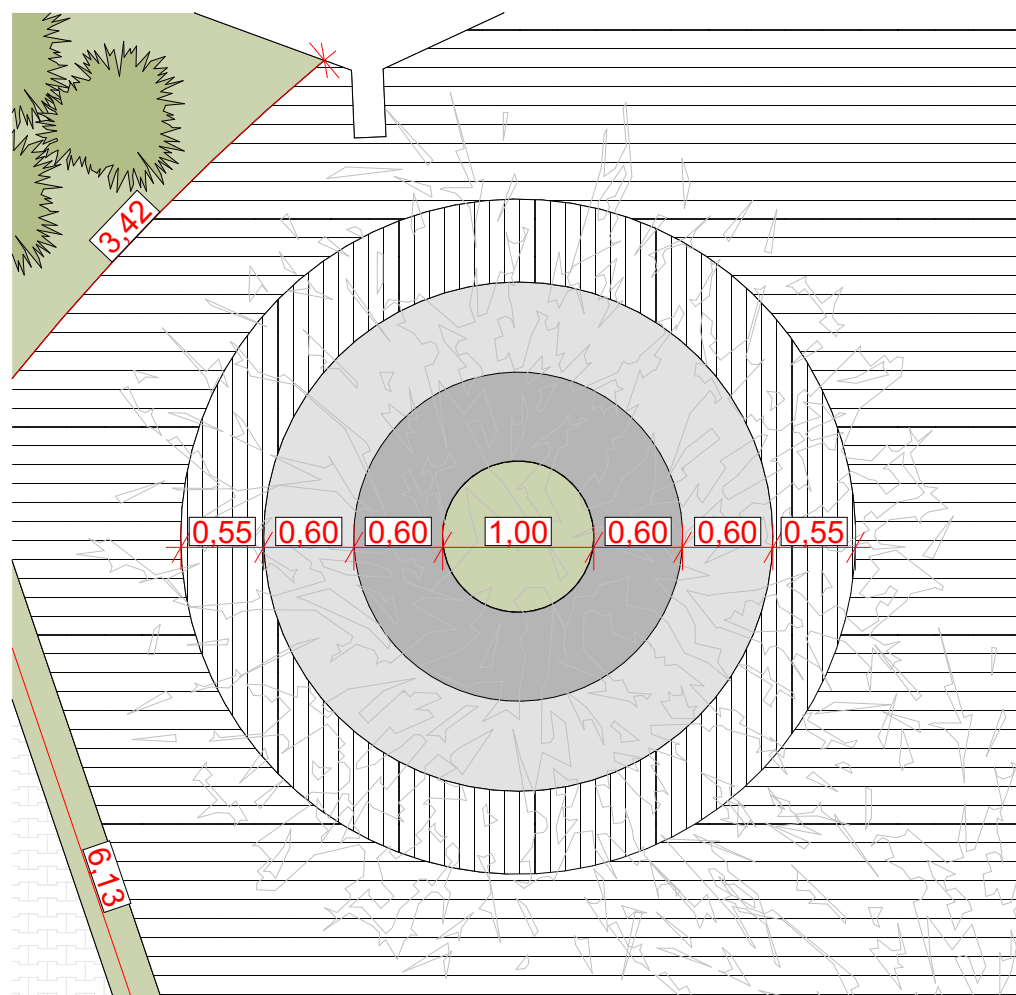
Planta Baixa Esc. 1:50
