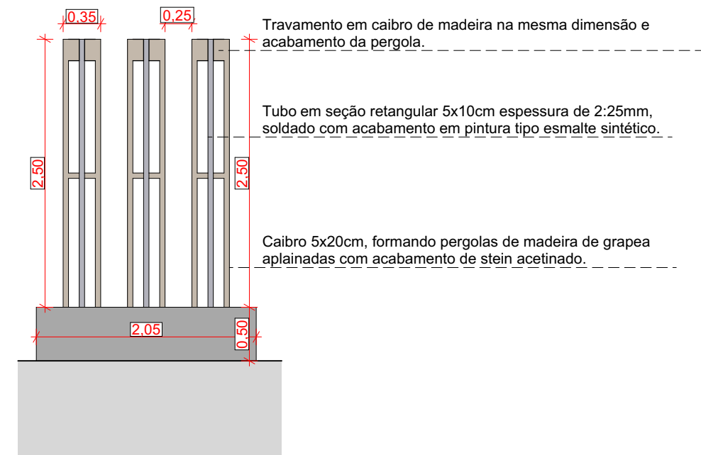
Elevação lateral Esc. 1:50
