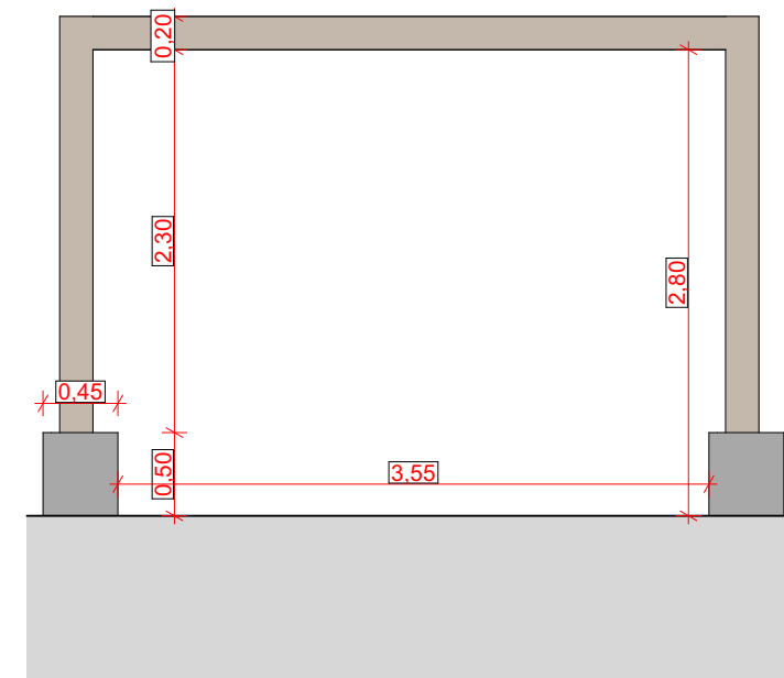
Elevação frontal Esc. 1:50
