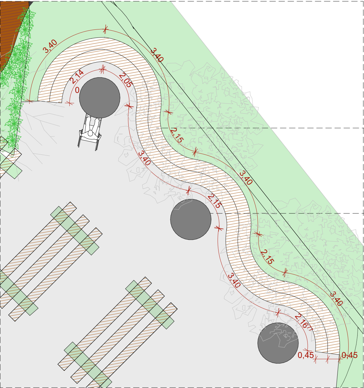
Planta Baixa Esc. 1:75
