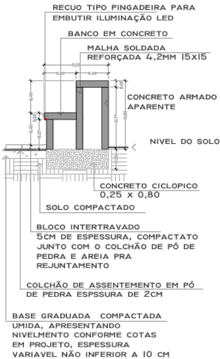
Detalhe Corte
