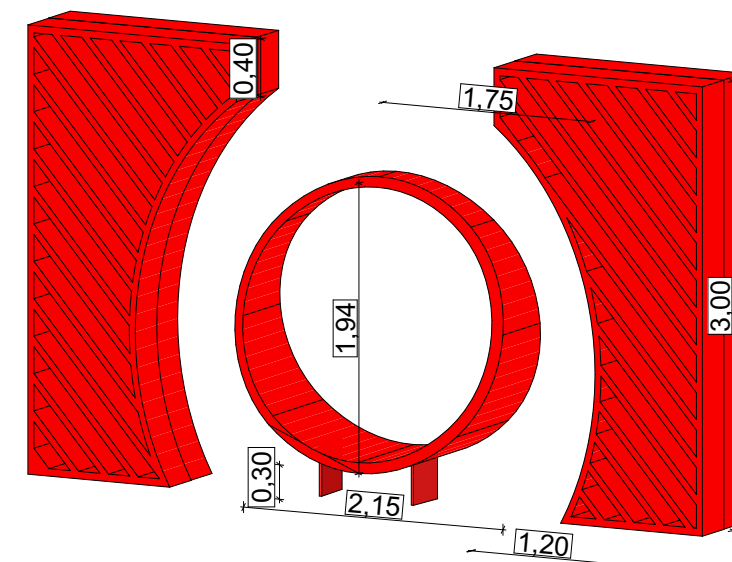
Detalhamento arco Esc. 1:50
