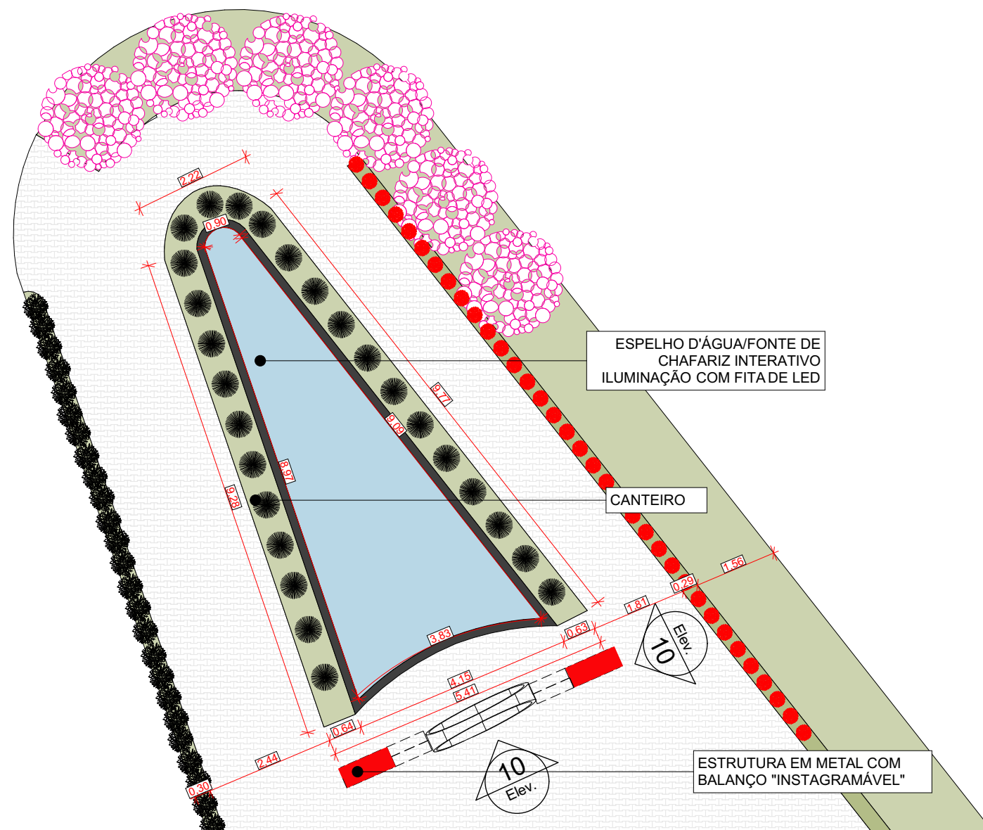
Planta Baixa Esc. 1:100
