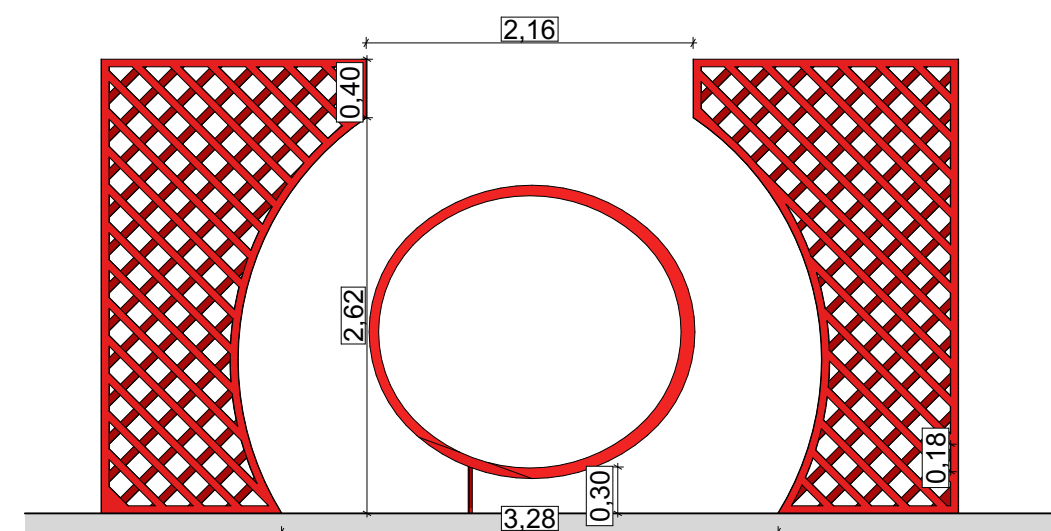
Elevação Esc. 1:50
