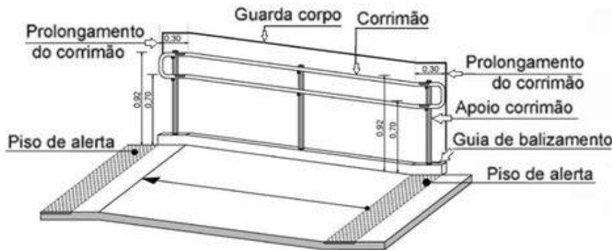
Figura 76 – Corrimãos em escada e rampa
