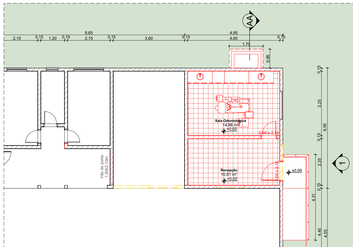
Planta de Reformas Esc. 1:100
