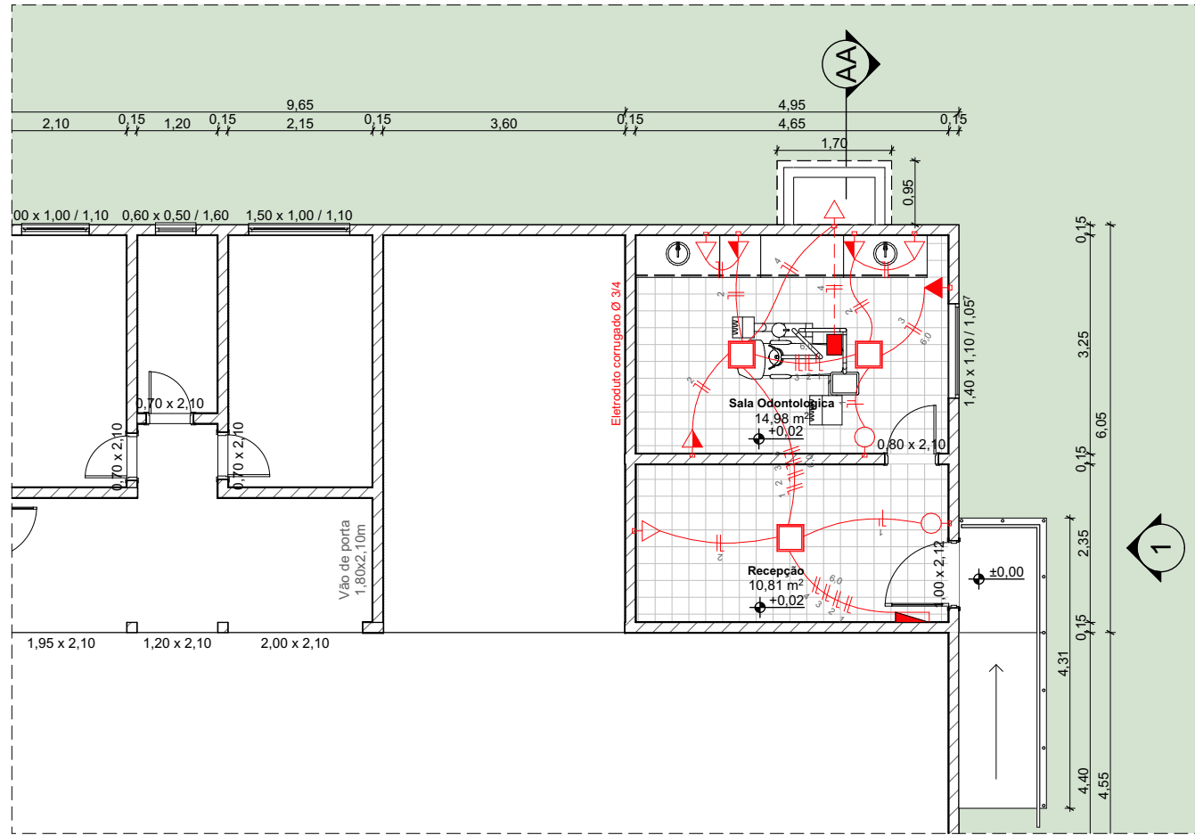
Planta Elétrica Esc. 1:100
