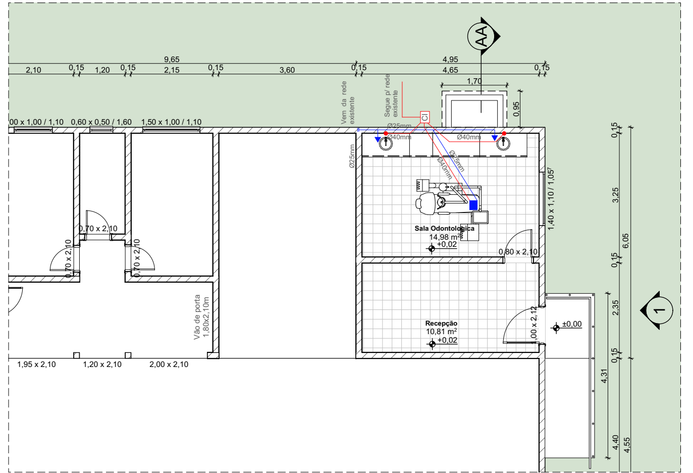
Planta de Hidrossanitário Esc. 1:100
