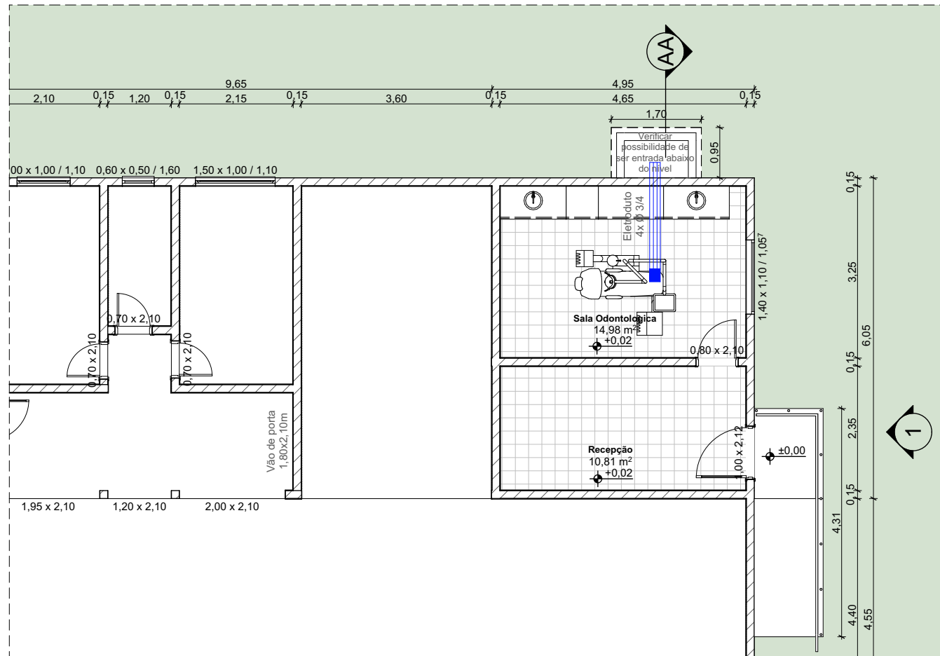
Planta de cadeira odontológica Esc. 1:100
