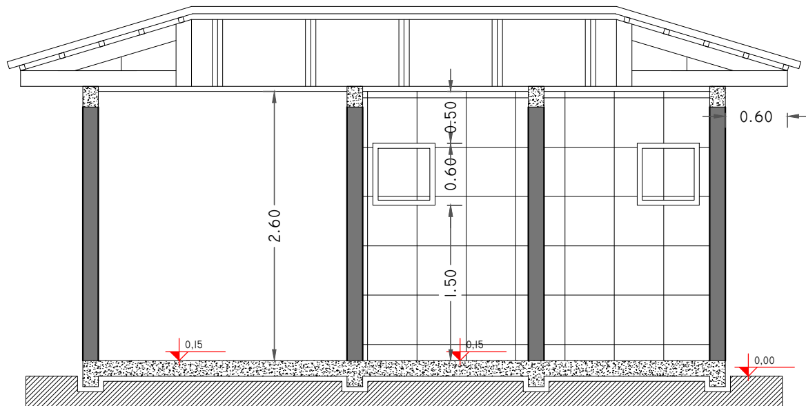
COORTE ESC: 1/50
