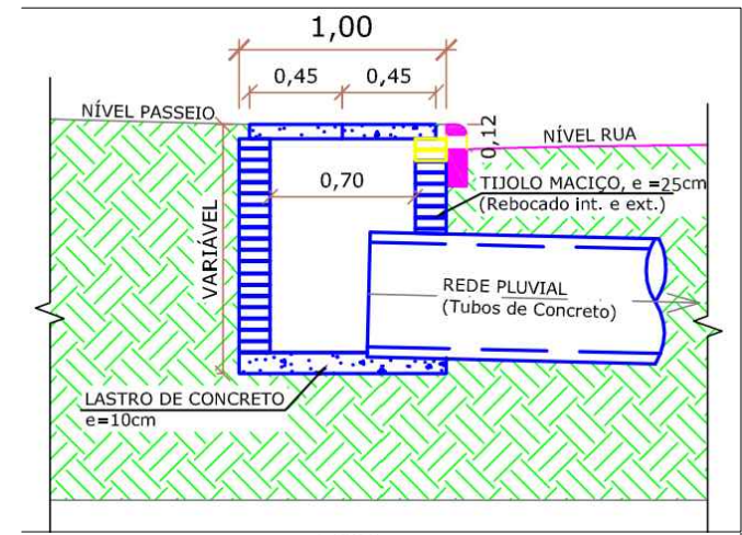
DETALHE BOCA DE LOBO
