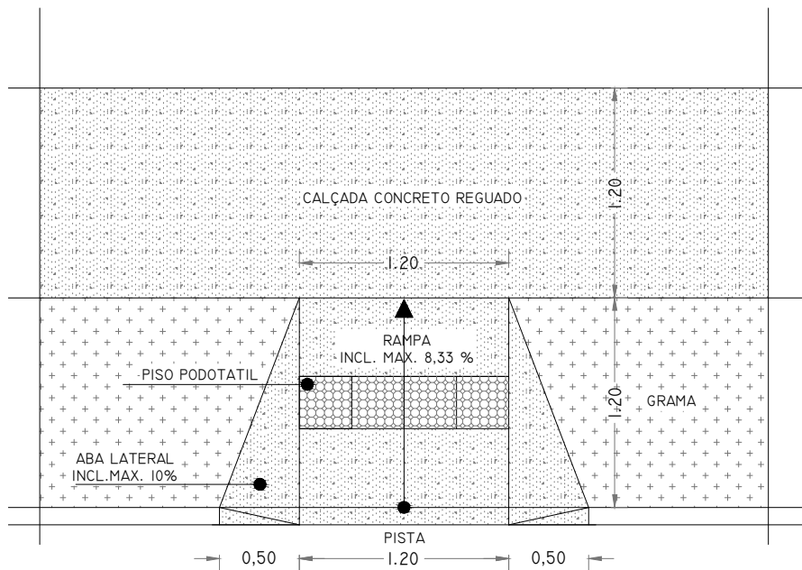
DETALHE RAMPA PNE ESCALA:
