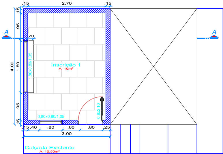
Planta Baixa Sub-solo Escala 1/75
