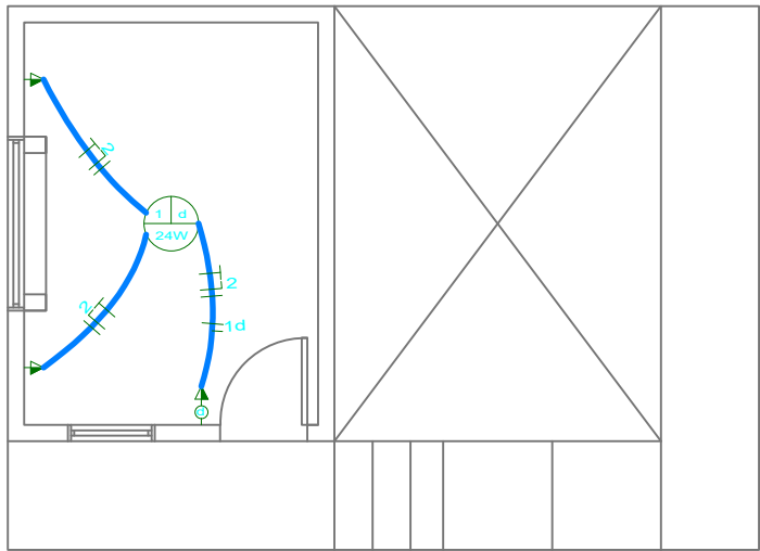
Projeto Elétrico Sub-solo Escala 1/75
