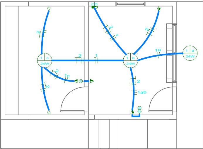
Projeto Elétrico Térreo Escala 1/75
