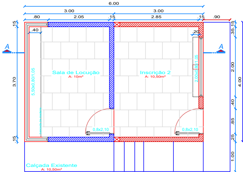
Planta Baixa Térreo Escala 1/75
