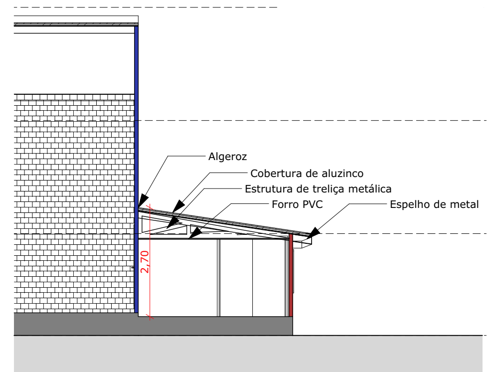
Corte AA
