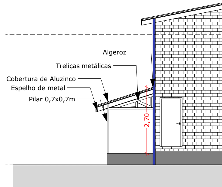
Corte BB
