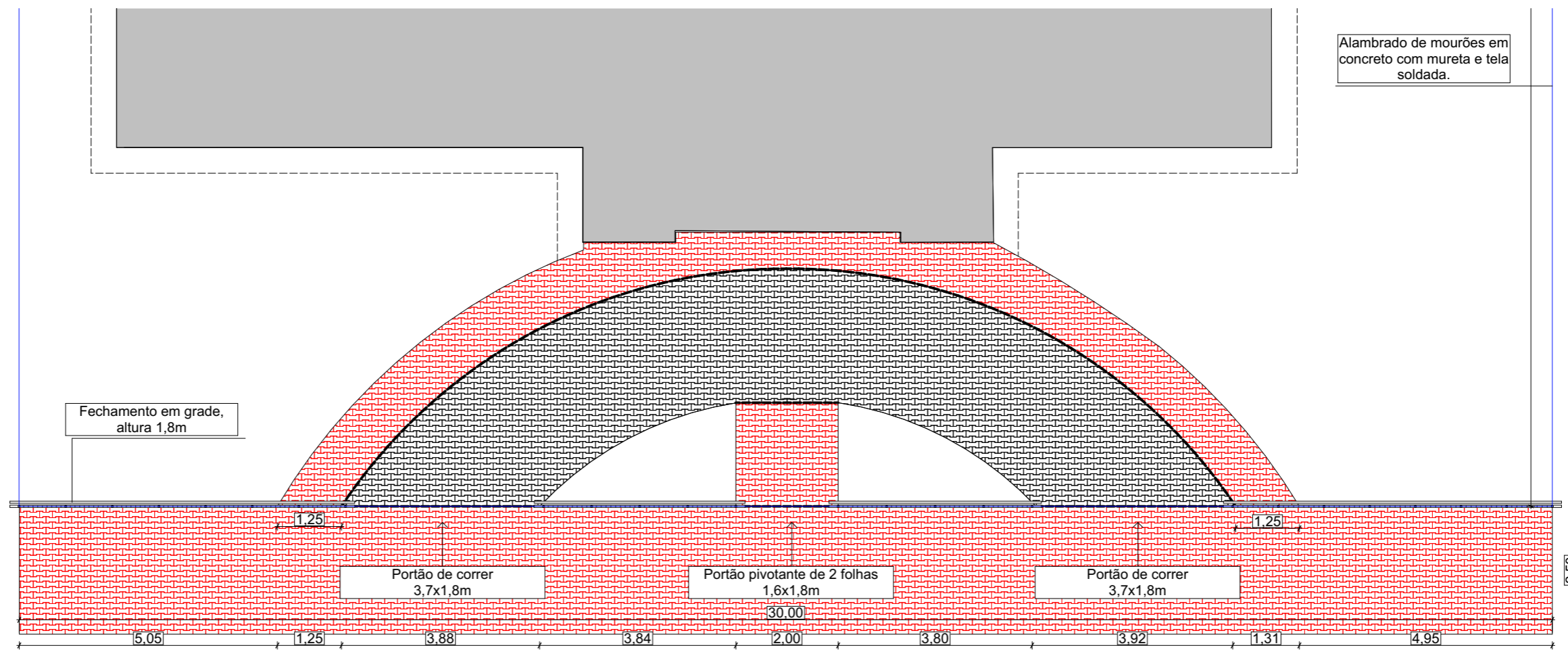
Planta Baixa Esc.1:150
