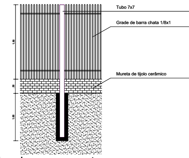
Detalhe do cercamento Esc.1:75
