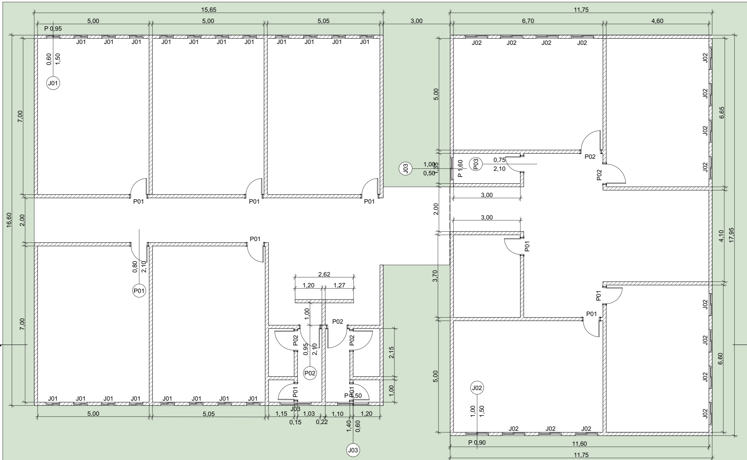
Planta Baixa Esc. 1:100
