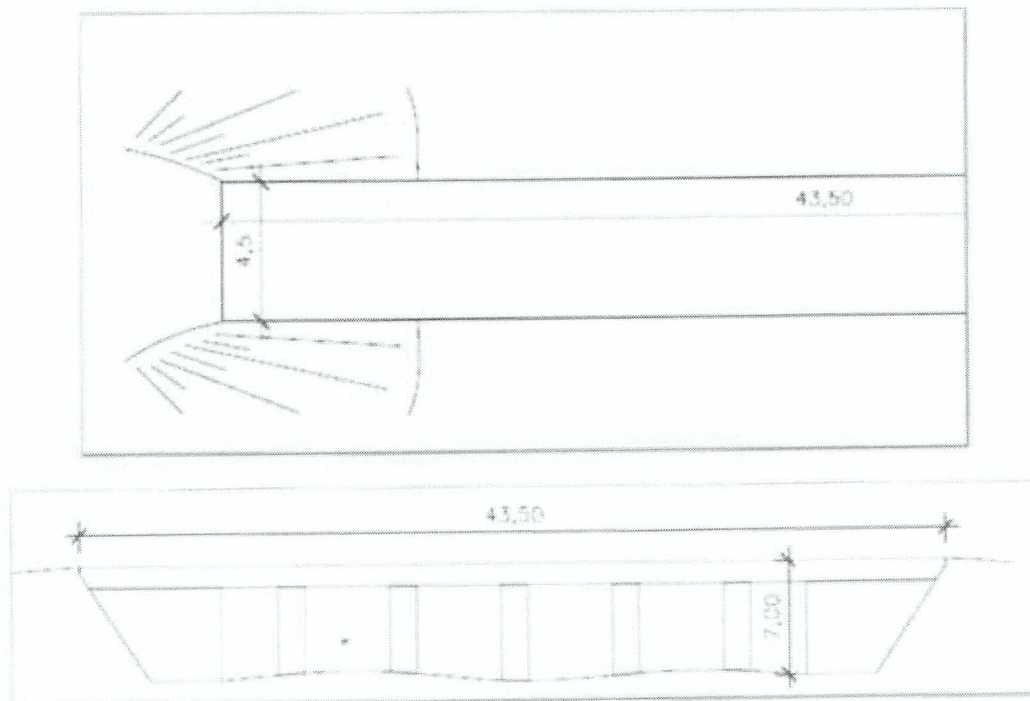
Figura 1 e 2 – Croqui Planta baixa e Perfil da Ponte
