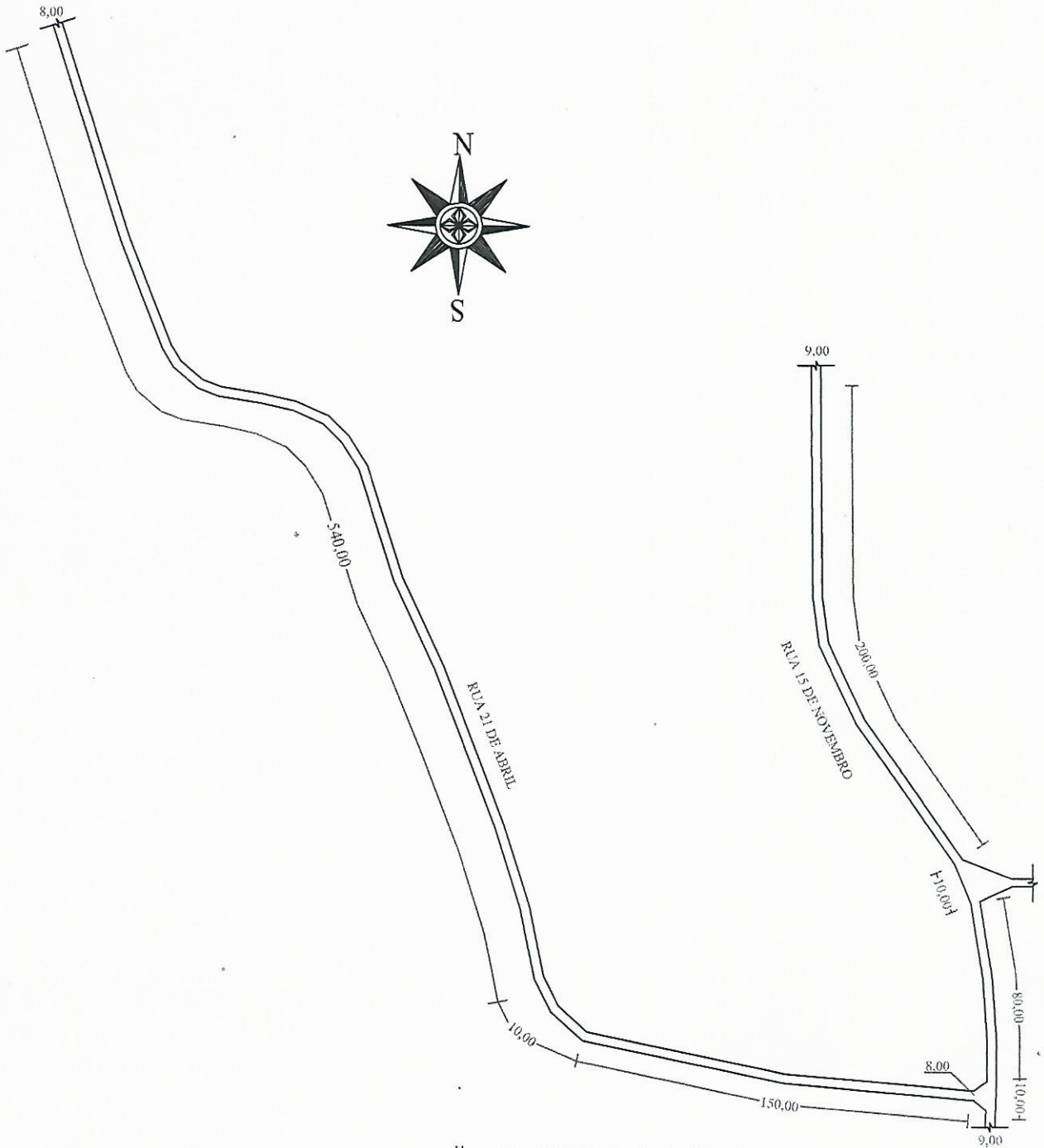
PLANTA BAIXA ÁREA TOTAL A SER PAVIMENTADA= 8.650,00 M 2
