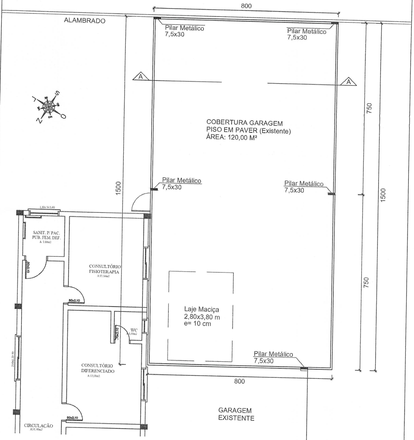
PLANTA BAIXA AMPLIAÇÃO
