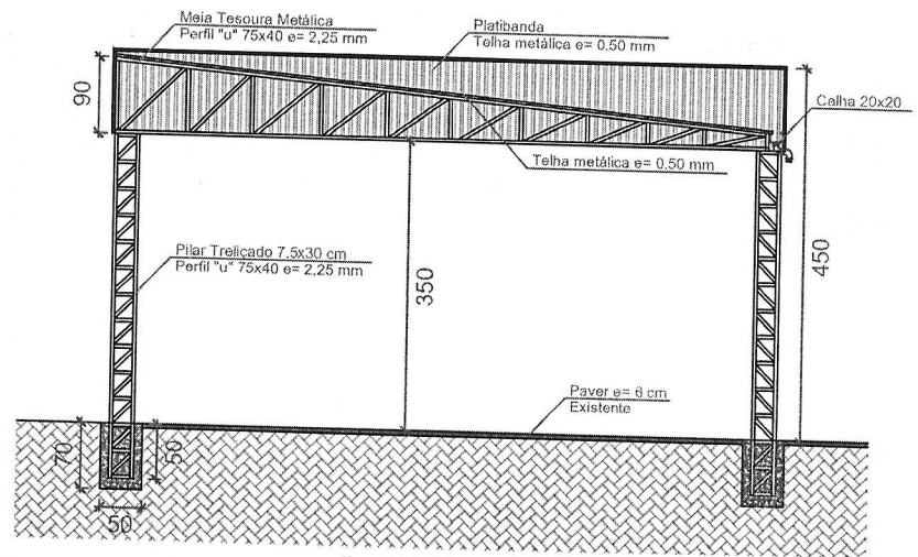
CORTE AA
