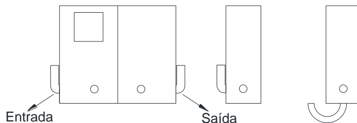
Caixa tipo III
