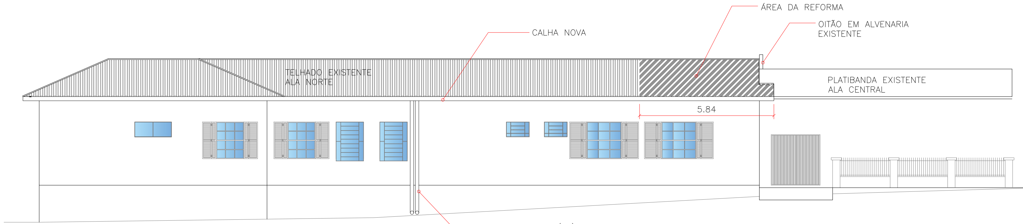
FACHADA NORTE Escala 1:150
