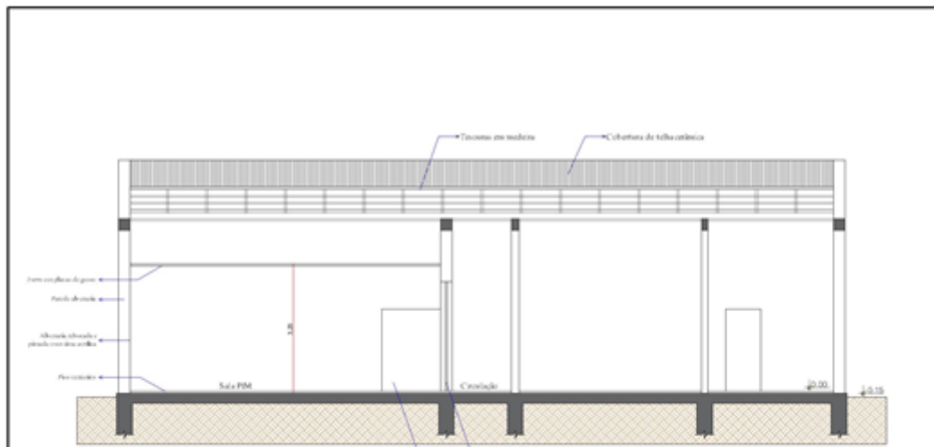
CORTE TRANSVERSAL Ese.: 1/125
