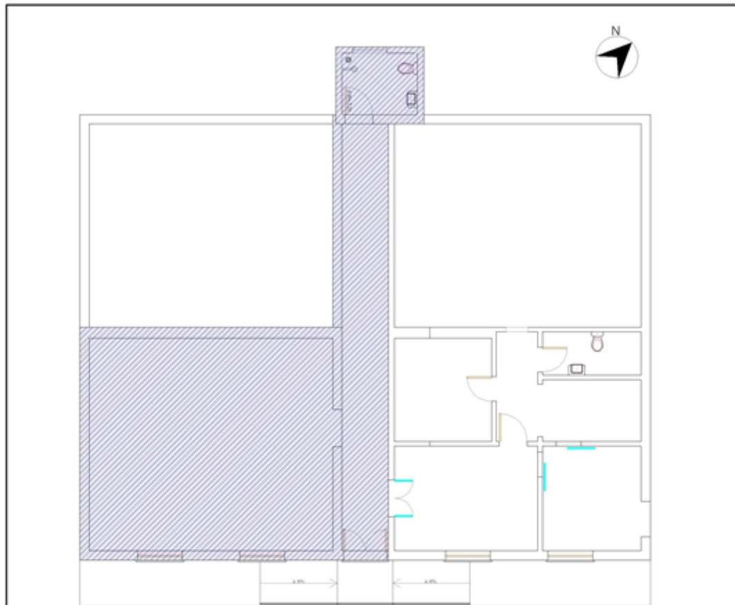
PLANTA BAIXA ÁREA A SER REFORMADA Área: 94,53m 2 Esc.: 1/125
