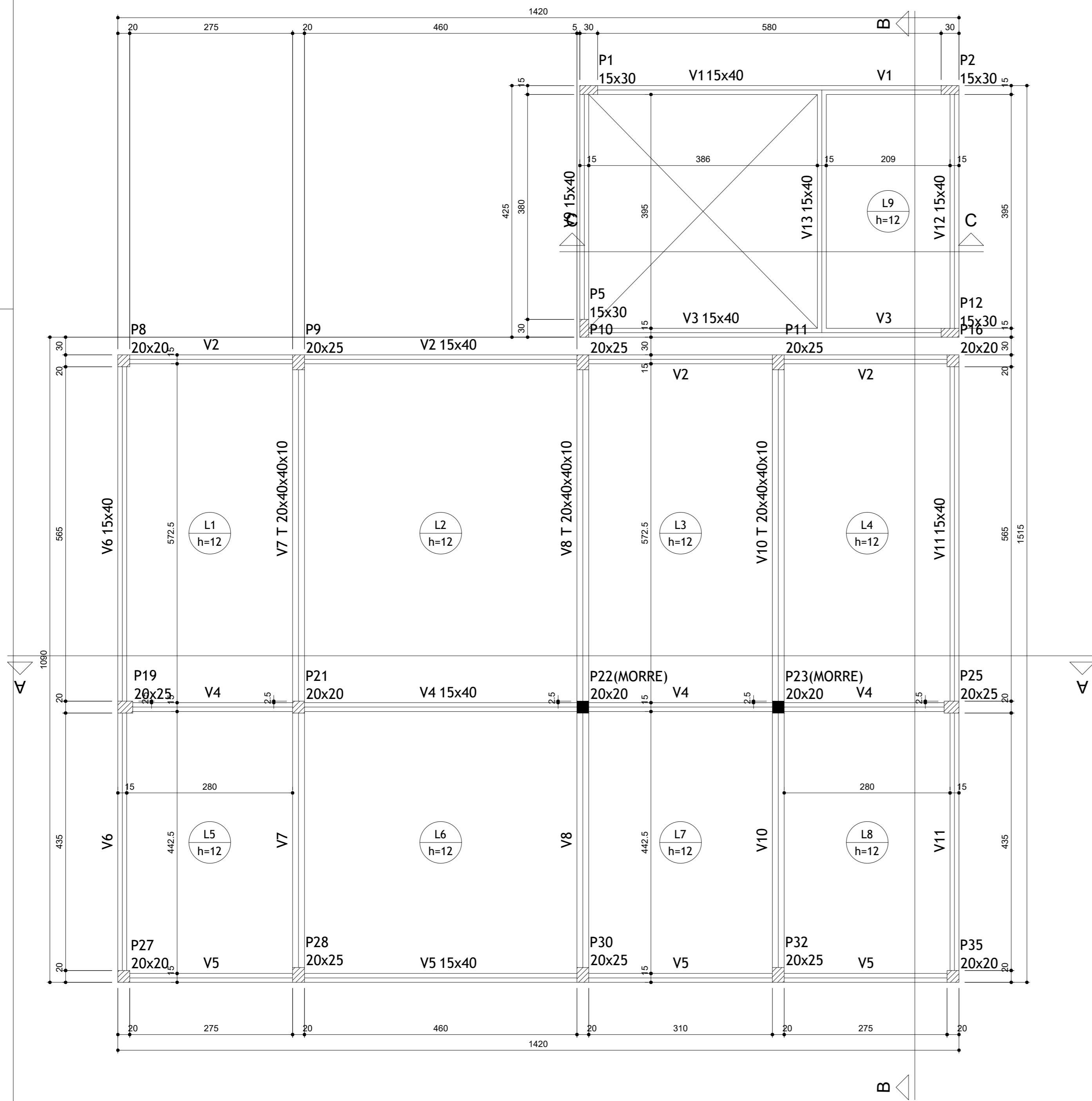
Forma do pavimento Pavimento 2 (Nível 365) escala 1:50
