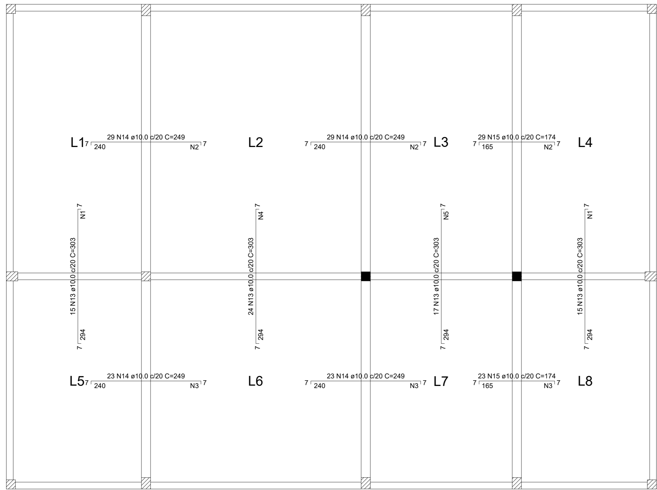
Armação negativa das lajes do pavimento Pavimento 2 escala 1:50
