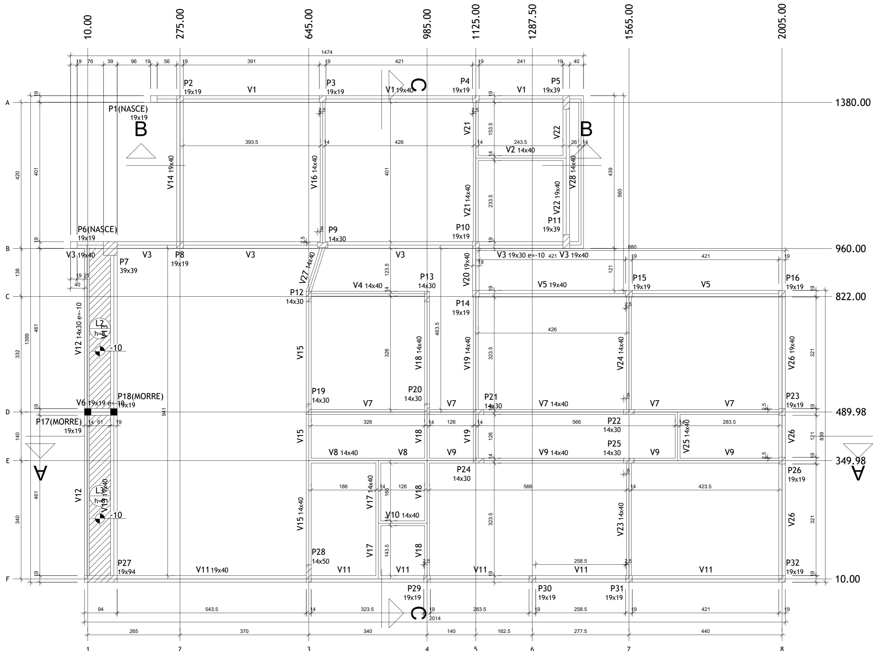
Forma do pavimento Pavimento - Térreo (Nível 0) escala 1:50
